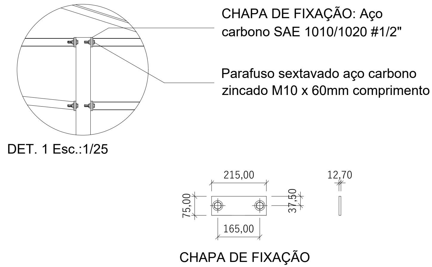
CHAPA DE FIXAÇÃO
