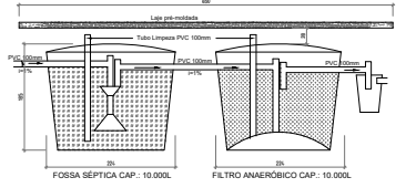
DETALHE FOSSA E FILTRO
