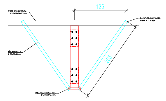
DETALHE MÃO-FRANCA
