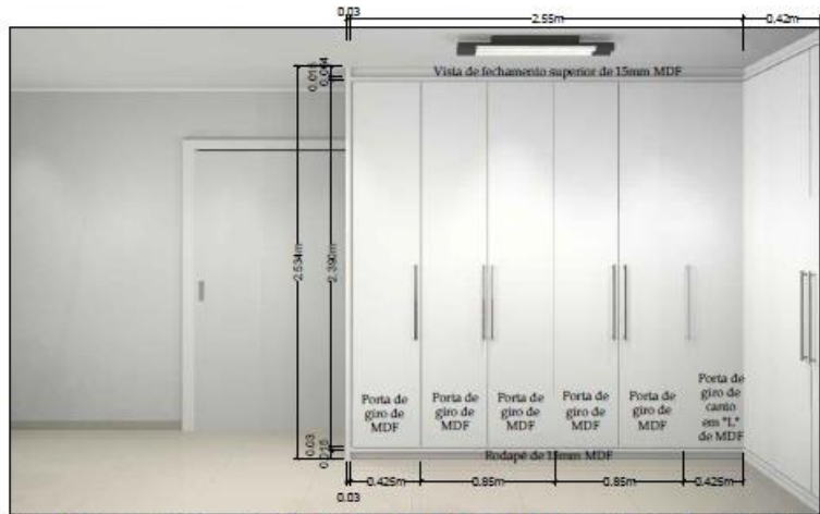
VISTA FRONTAL B MÓVEL SALA DAS PROFESSORAS O1
