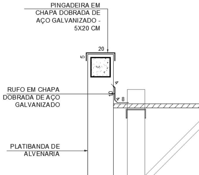
Figura 8 – imagem exemplificativa de detalhe de rufo/alvenaria e pingadeira
