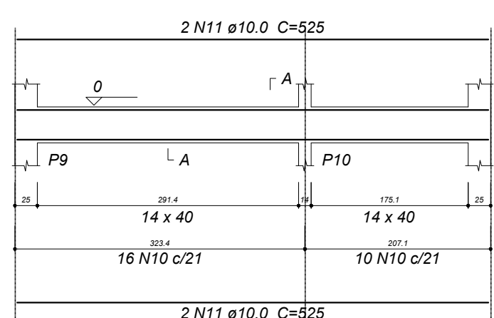
V4 ESC 1:30
