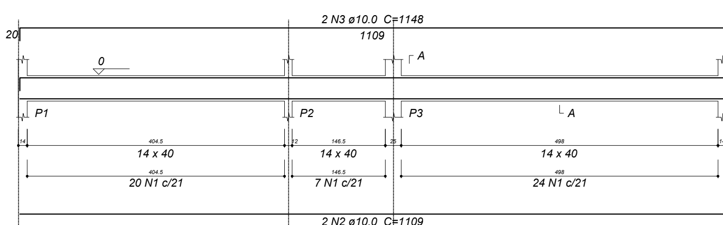
V9 ESC 1:30
