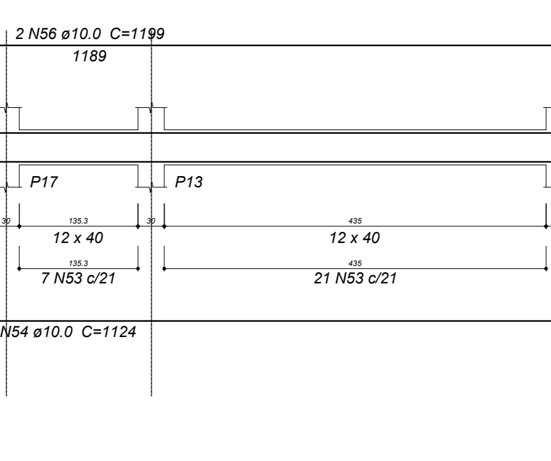
V30 ESC 1:30
