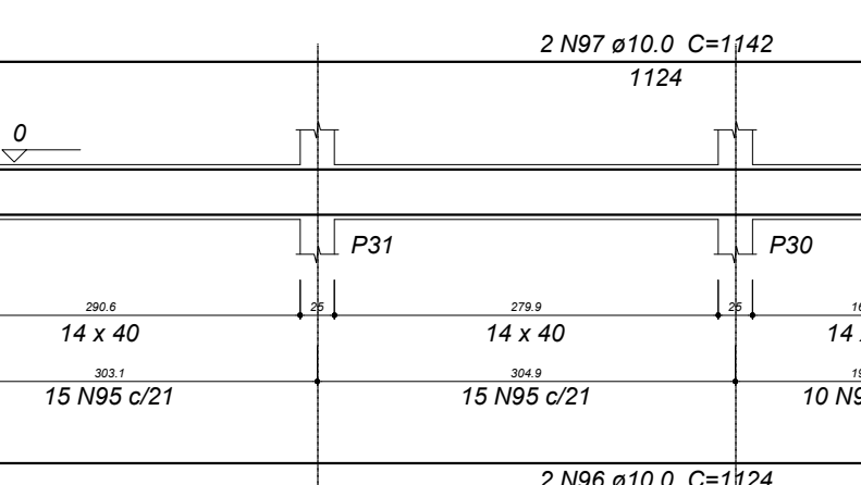
V31 ESC 1:30
