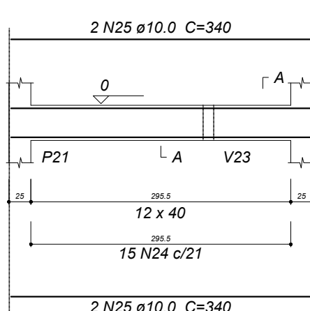
V9 ESC 1:30
