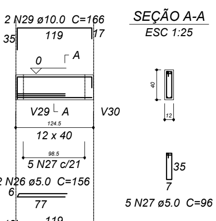
V10 ESC 1:30
