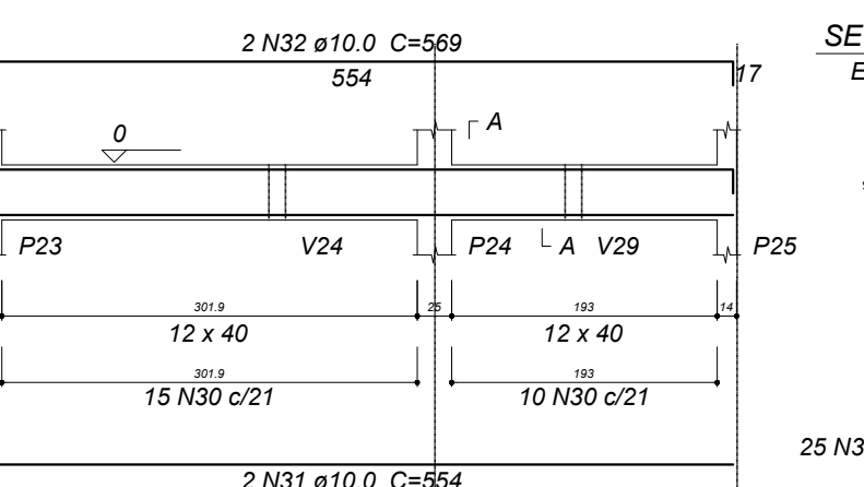
V11 ESC 1:30
