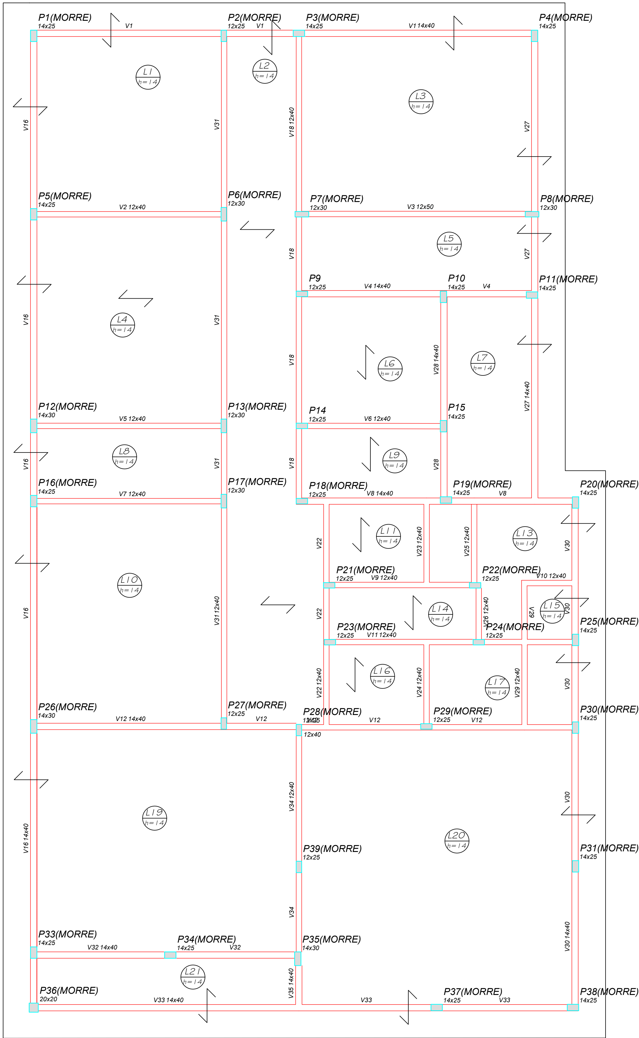
Forma do pavimento Térreo escala 1:50
