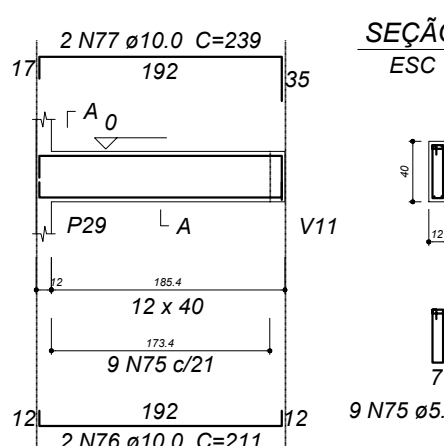
V25 ESC 1:30
