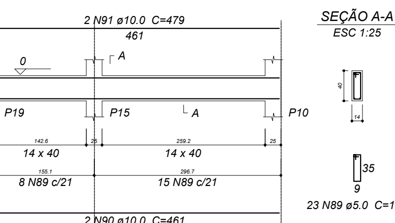
V29 ESC 1:30
