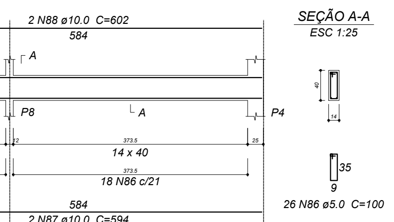
V28 ESC 1:30
