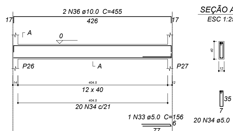
V12 ESC 1:30
