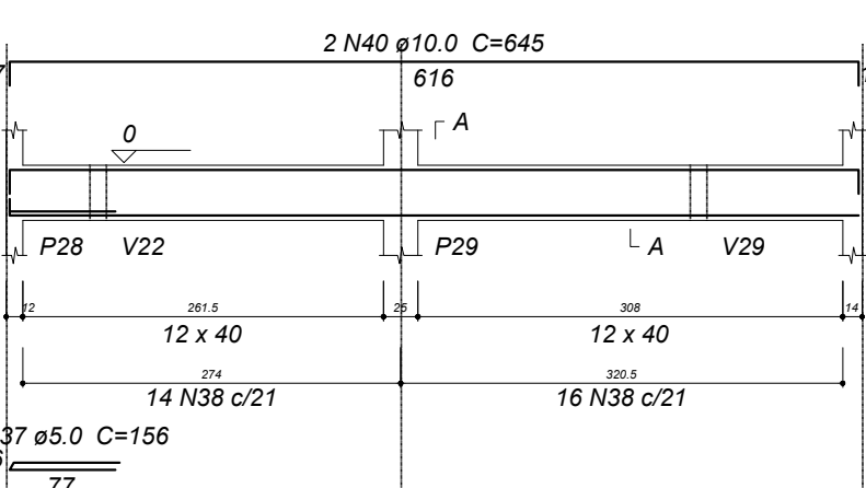
V13 ESC 1:30
