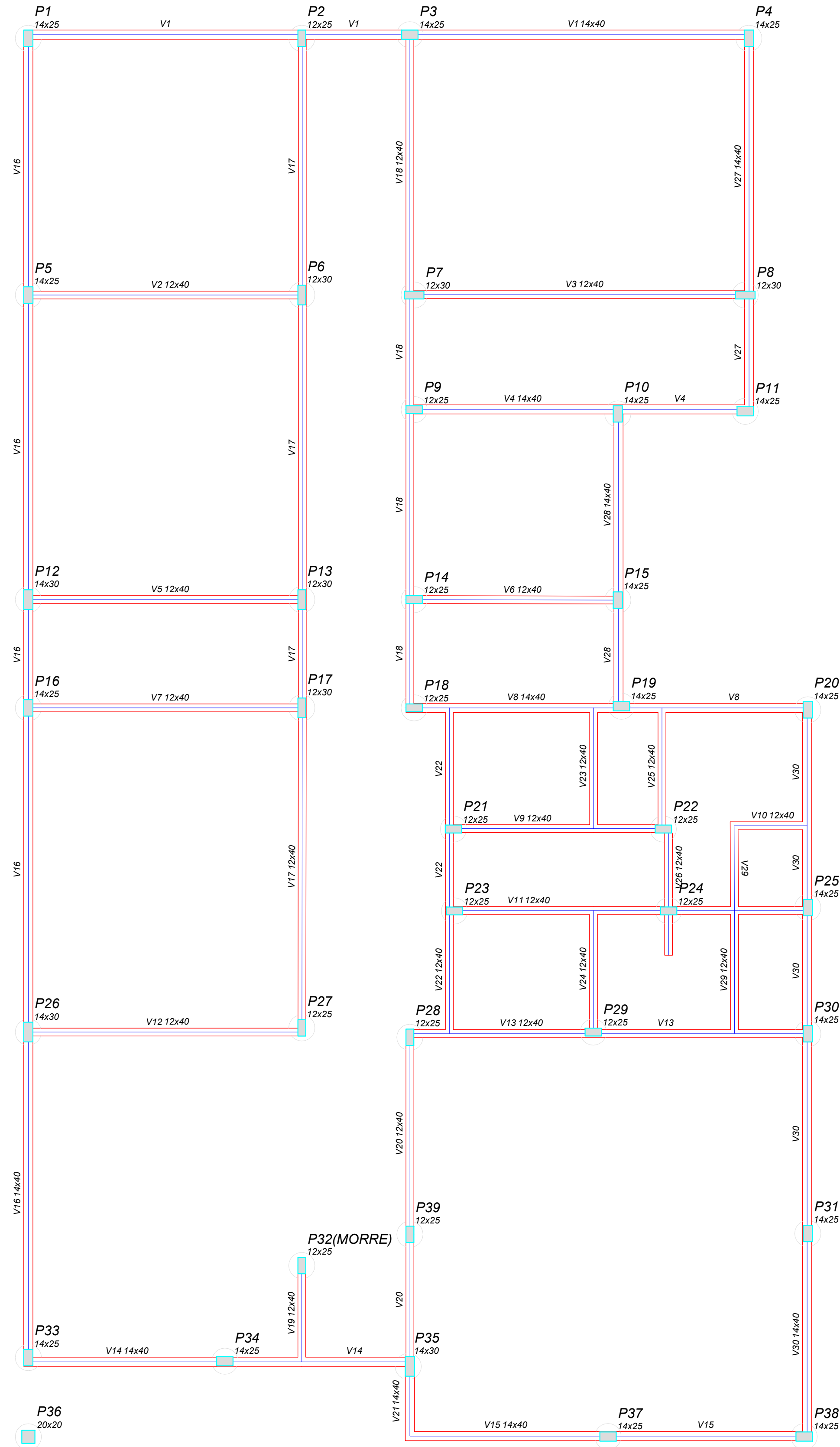
Forma do pavimento Fundação escala 1:50
