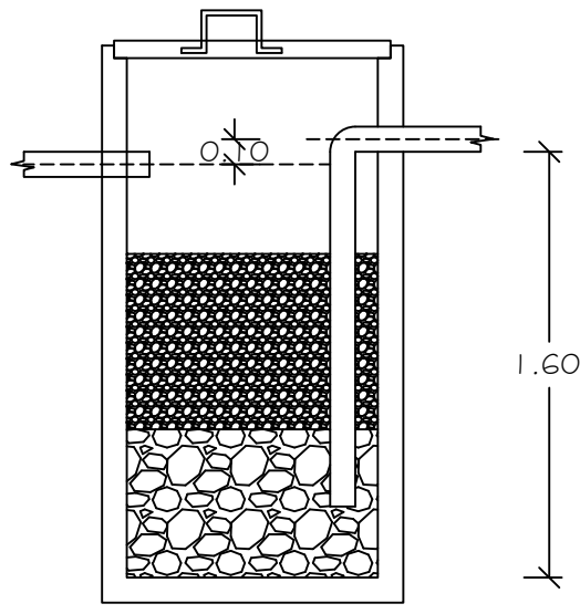
Corte
