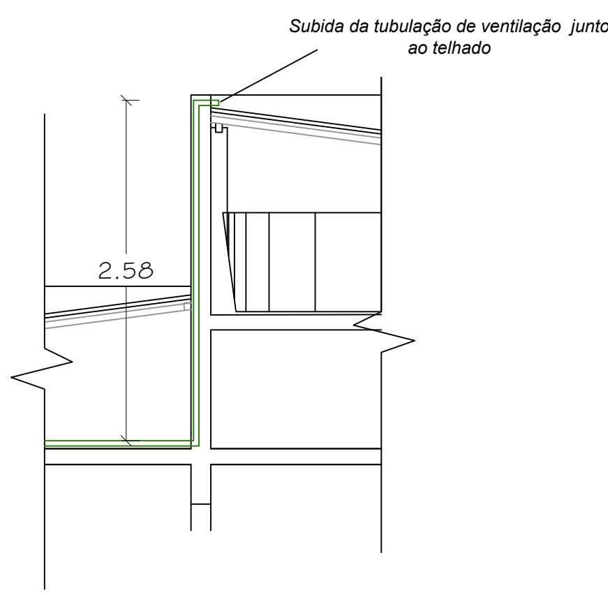
Detalhe 1
