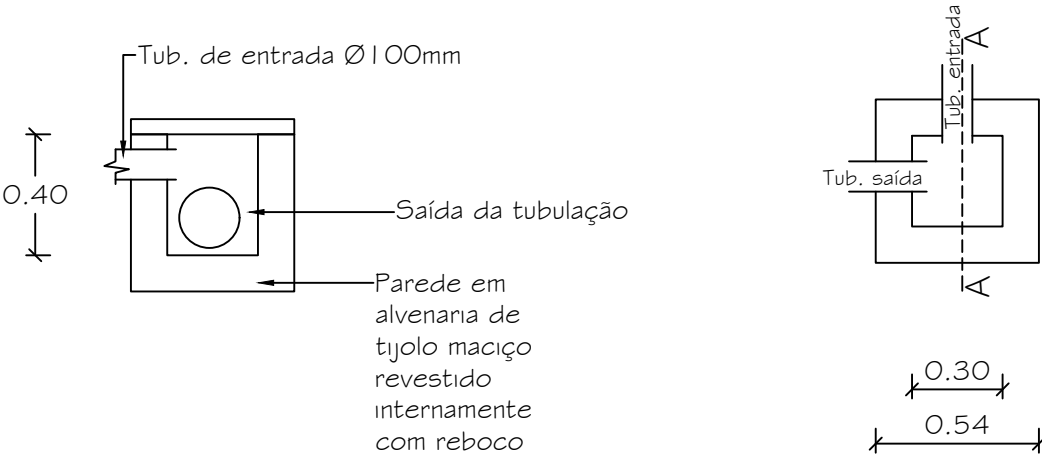
Caixa de passagem/areia
