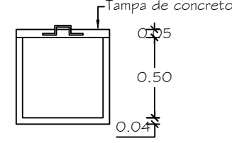
Corte
