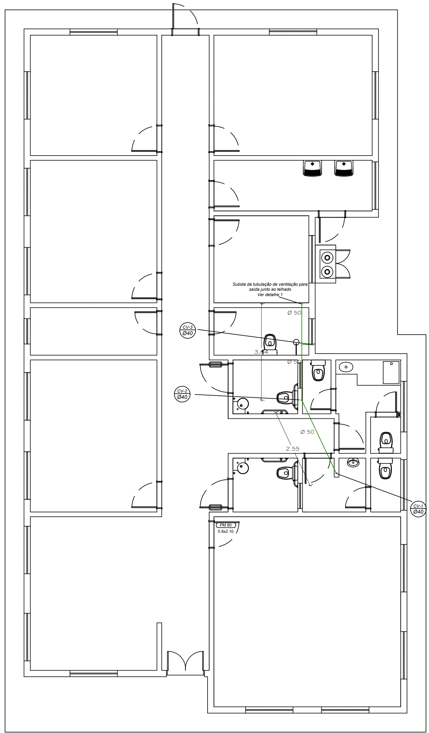
Planta Baixa de Instalações Hidrossanitárias de Esgoto - Tubulação de Ventilação Escala 1:75
