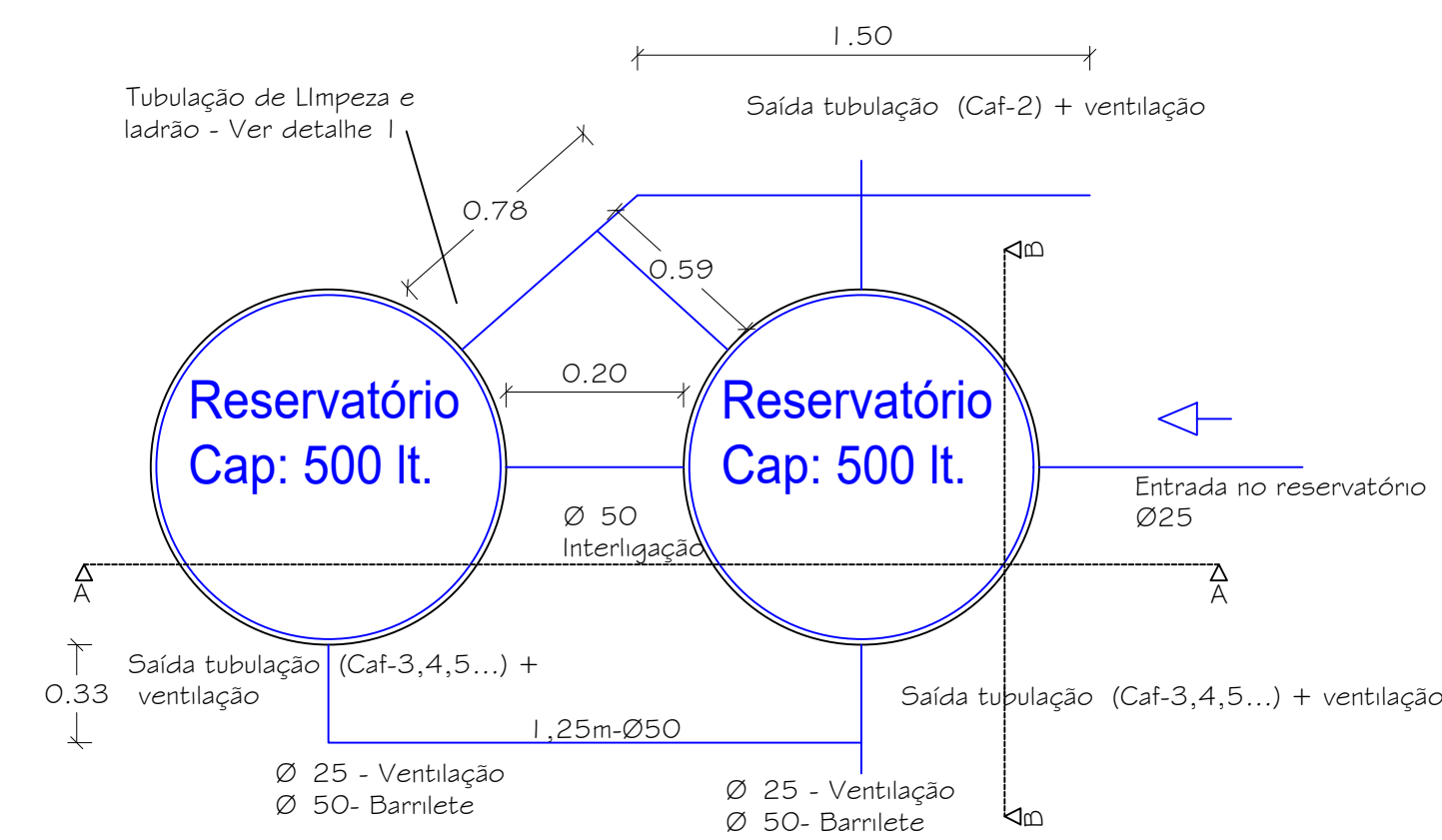
Planta Baixa dos Reservatórios
