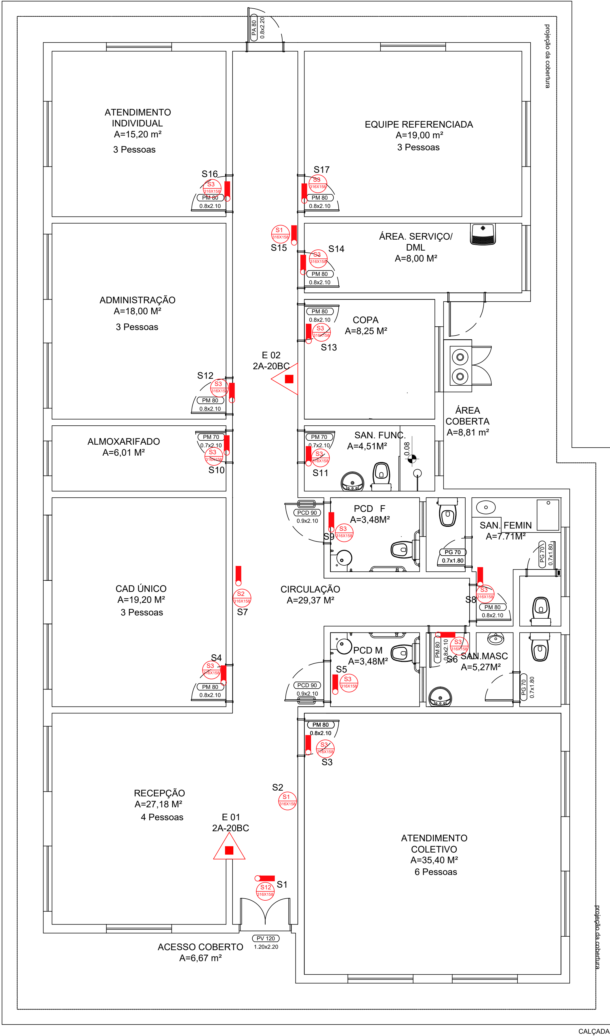
Planta Baixa de Instalações de Prevenção Contra Incendio Escala 1:50
