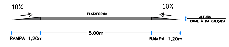
SEÇÃO TRANSVERSAL DA FAIXA ELEVADA
