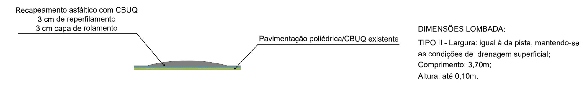
SEÇÃO TRANSVERSAL DA LOMBADA Ondulação Transversal ou Lombada executada em CBUQ
