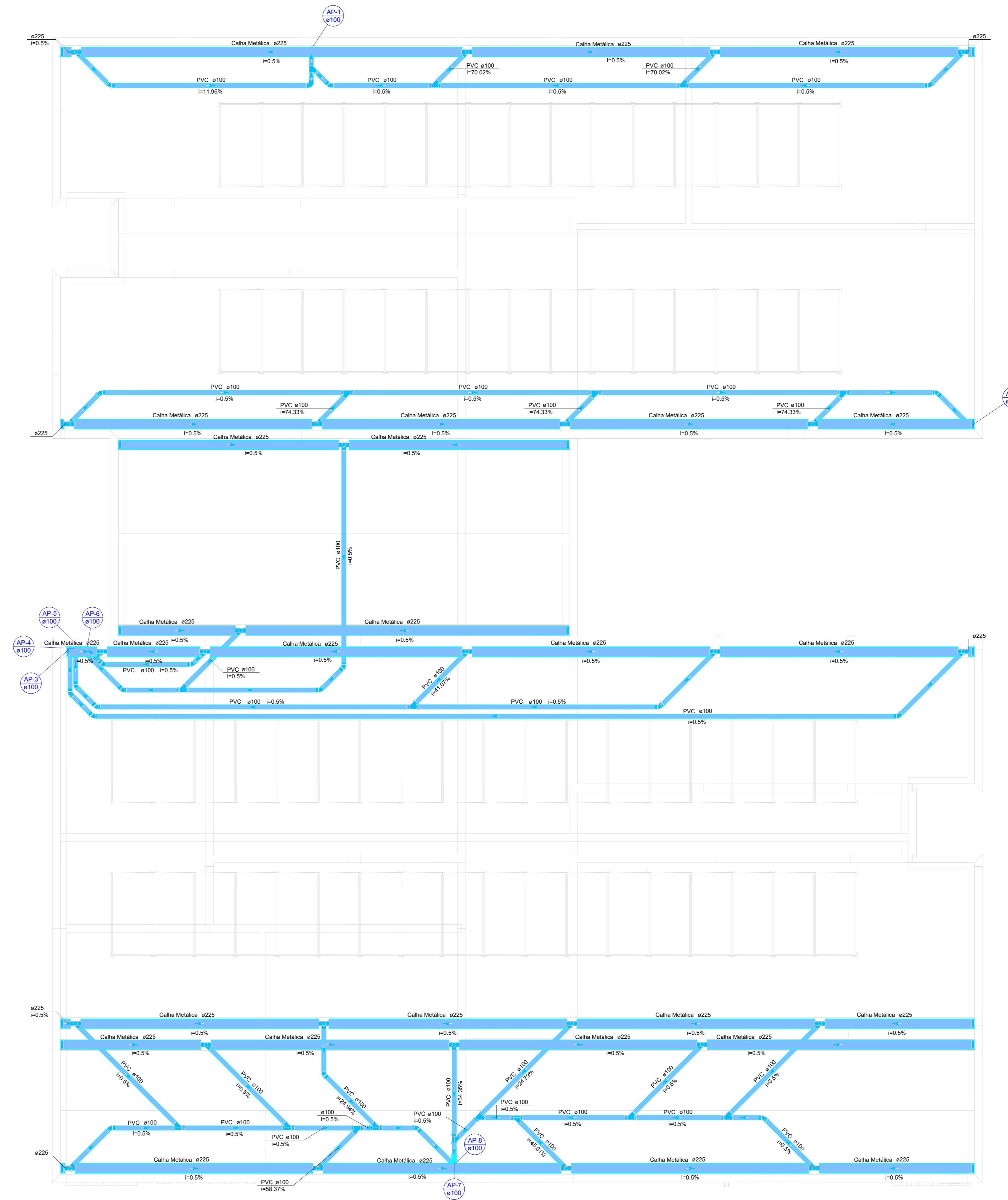
PLANTA - SANITÁRIO - COBERTURA ESC. 1/50
