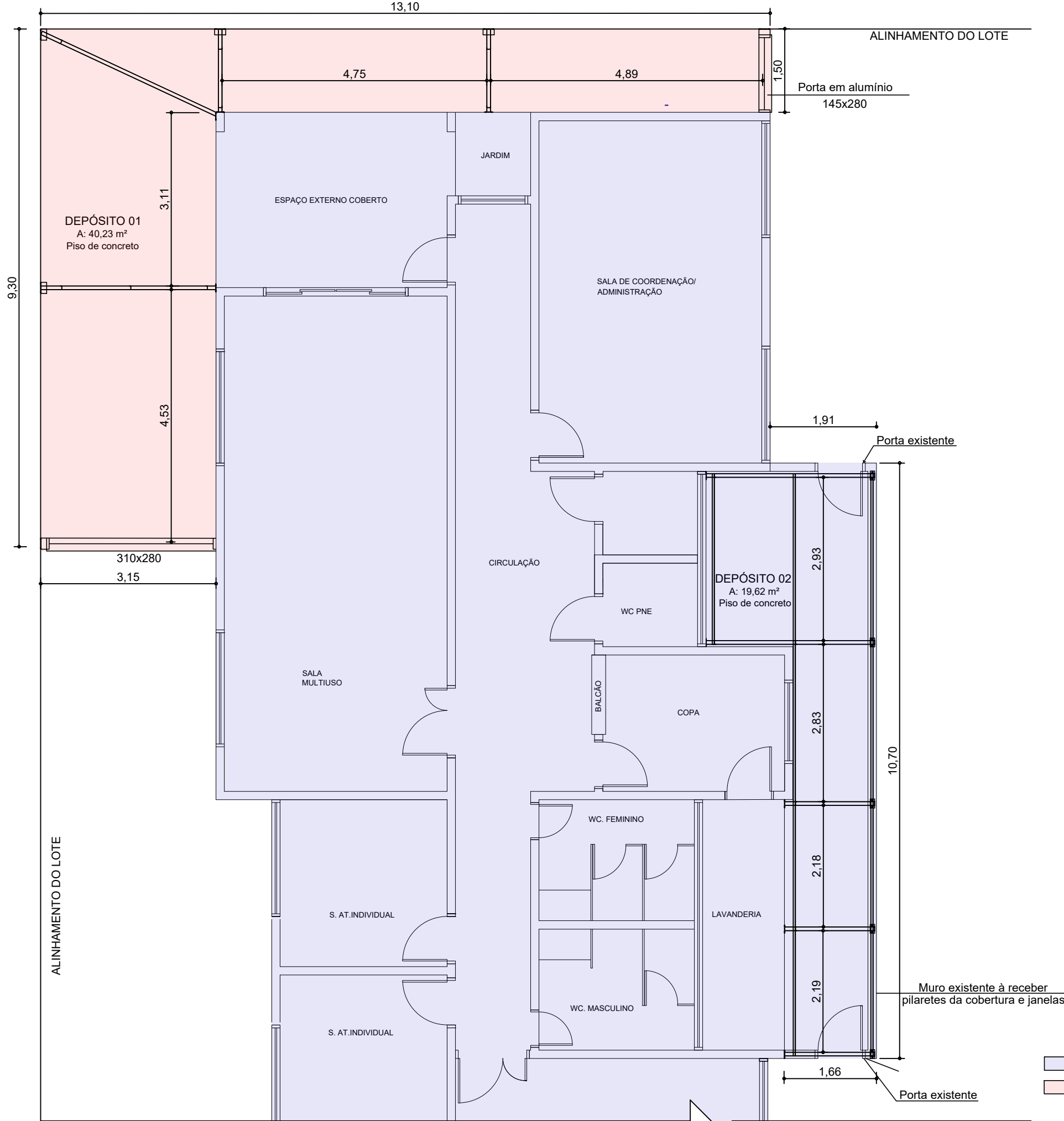
PLANTA BAIXA A: 66,42 m² ESC. 1/75
