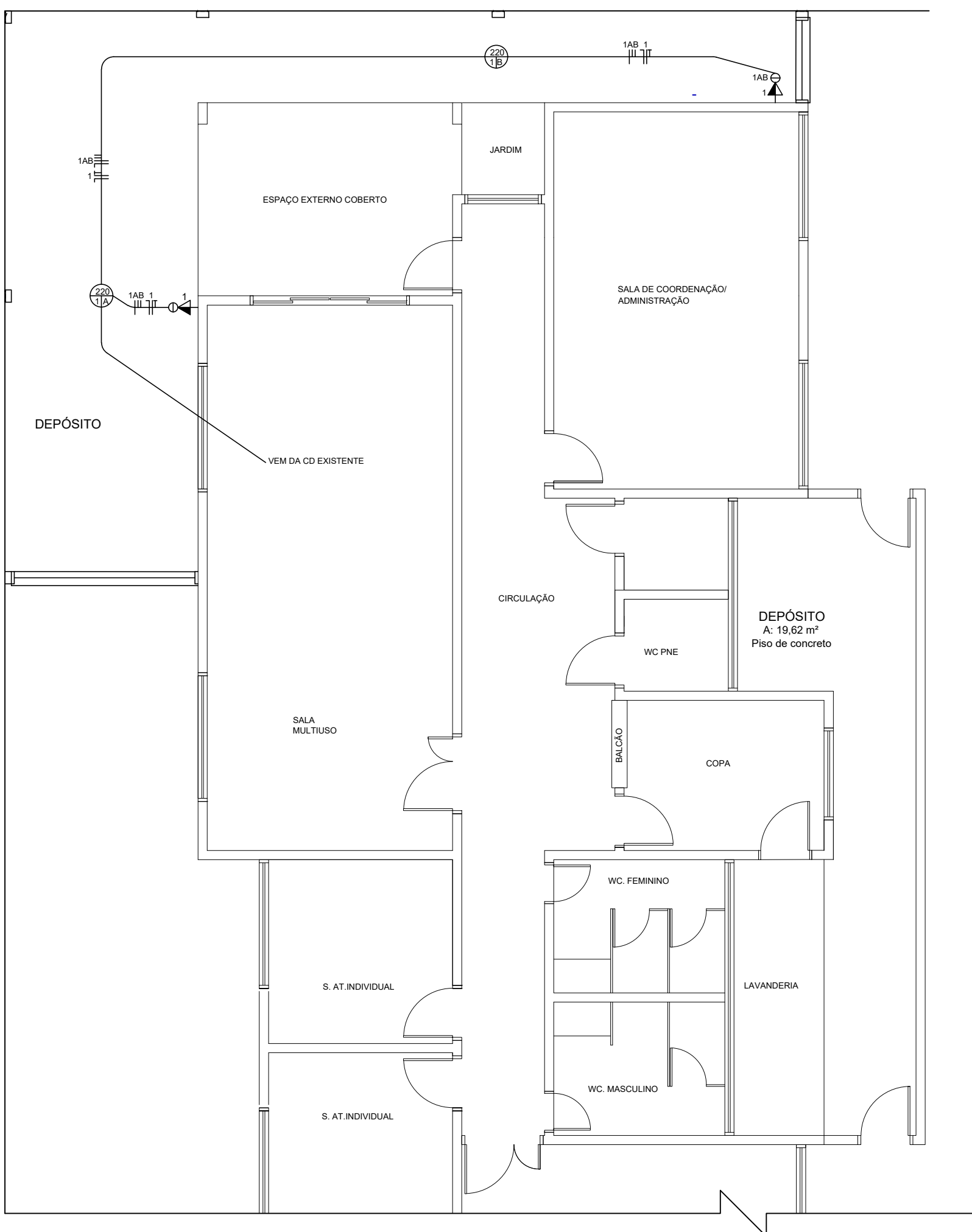
ELÉTRICO - PLANTA BAIXA ESC. 1/75
