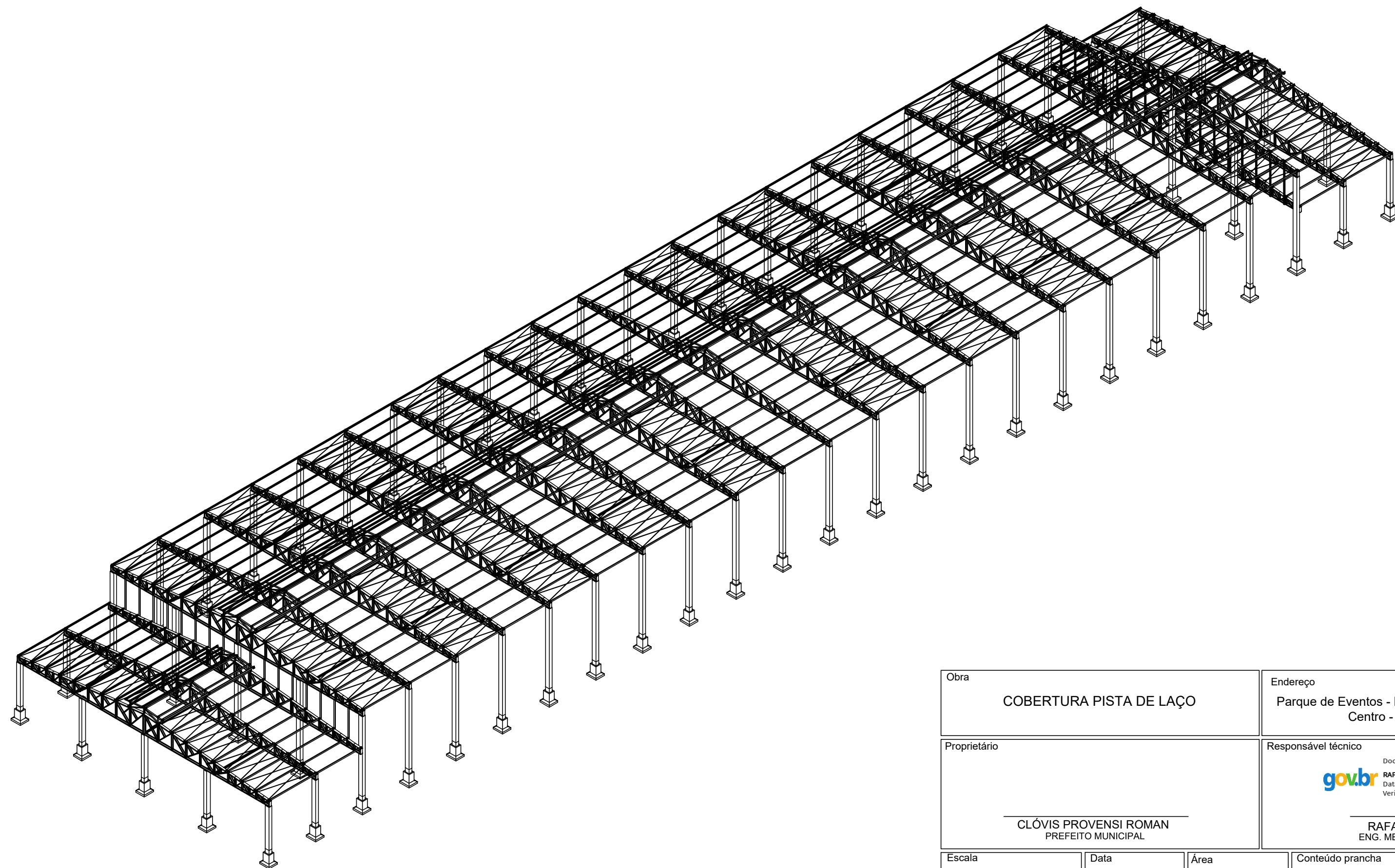
REPRESENTAÇÃO 3D DA ESTRUTURA SEM ESCALA
