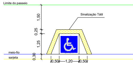
Detalhe - Rampa de Acessibilidade - 2 Un. Sem Escala
