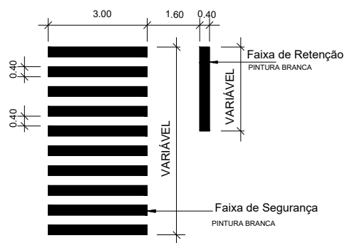
Detalhe - Faixa de Segurança e Retenção Sem Escala
