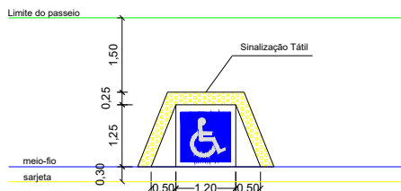
Detalhe - Rampa de Acessibilidade - 2 Un. Sem Escala
