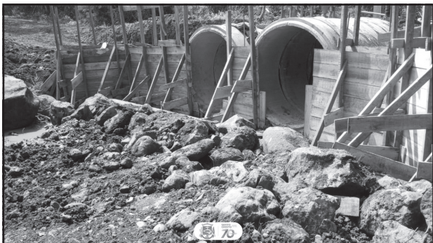
Confecção das caixas para a concretagem de ponte baixa em linha Orion
