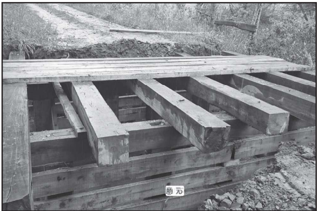
Construção de ponte na Linha Júpiter.
