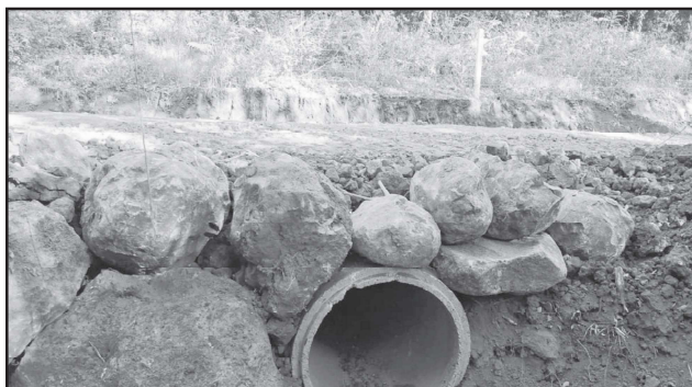
Construção de tubulação na Linha Rolador Baixo
