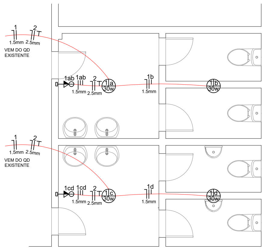
PLANTA ELÉTRICO Esc. 1/50
