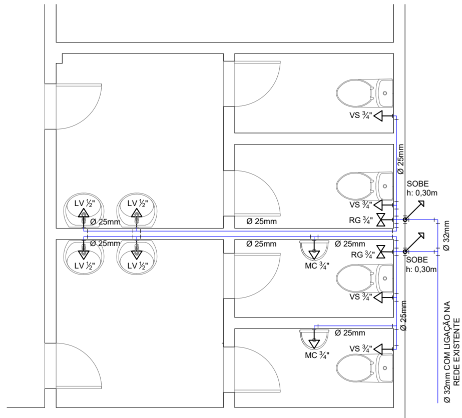
PLANTA HIDRÁULICO Esc. 1/50
