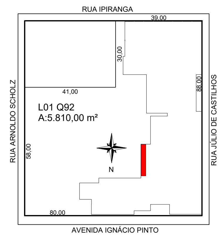
PLANTA DE LOCALIZAÇÃO ESC 1:1000
