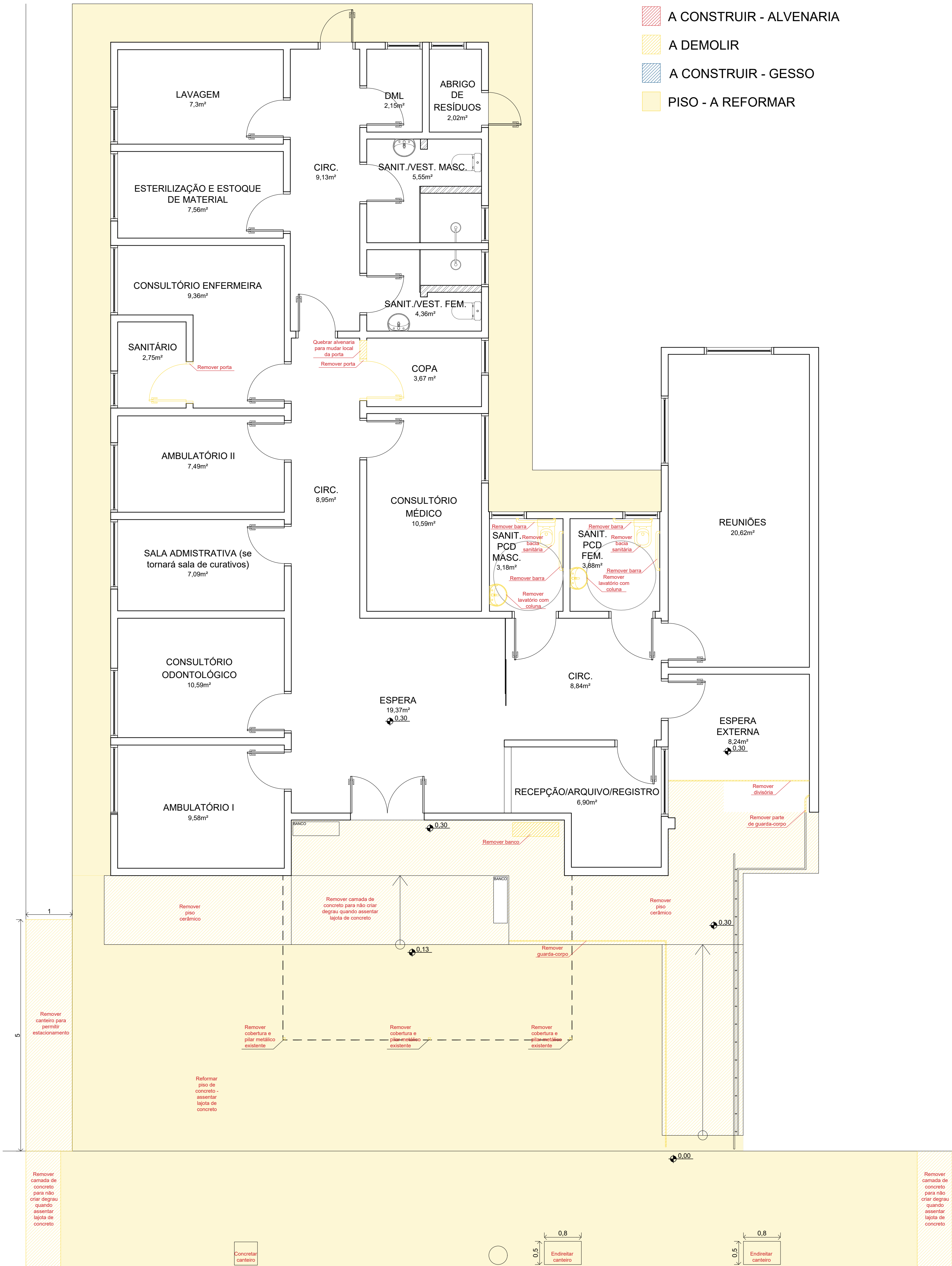
PLANTA BAIXA - A DEMOLIR ESC 1/50 Área: 202,62m²
