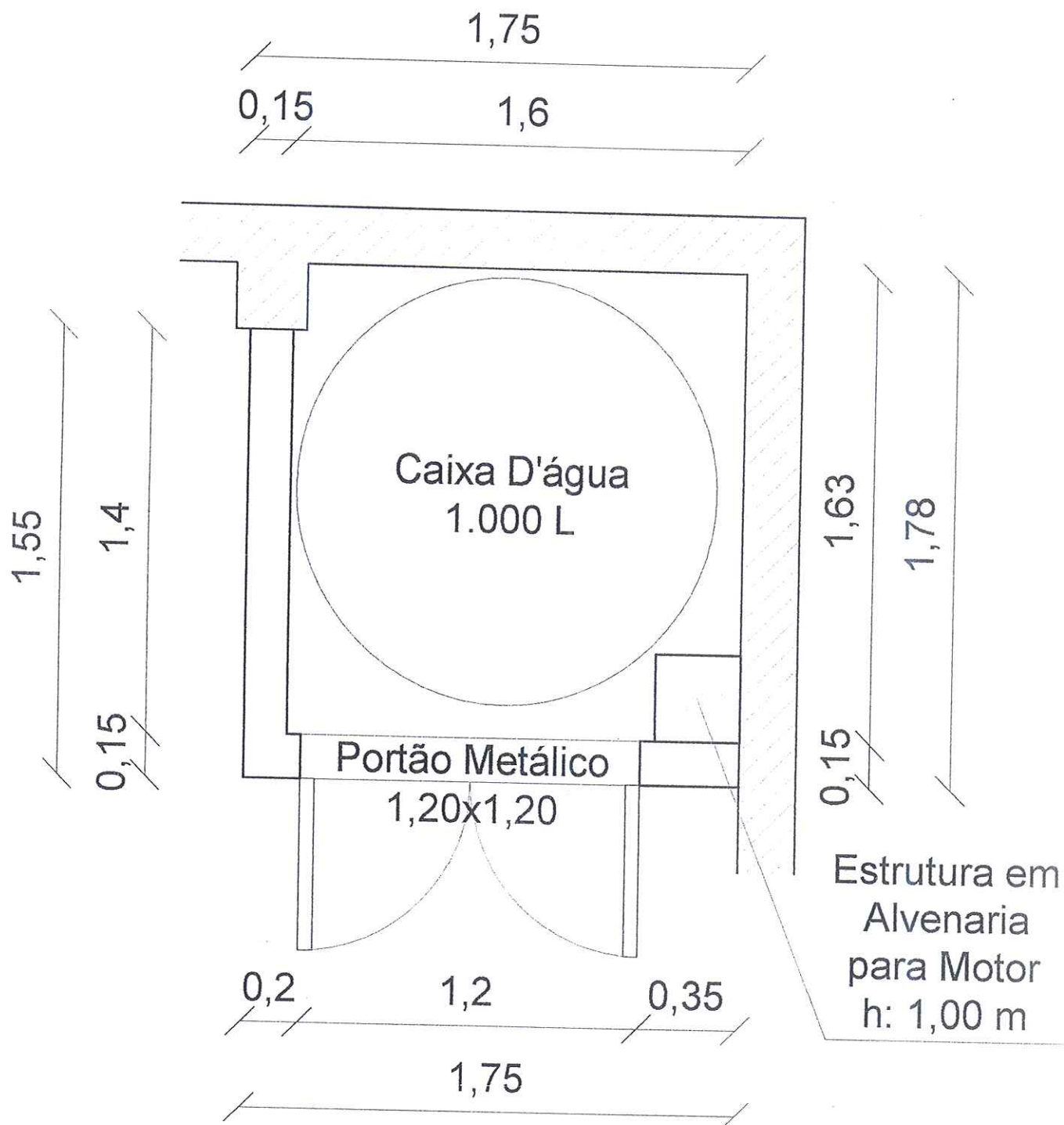
PLANTA BAIXA
