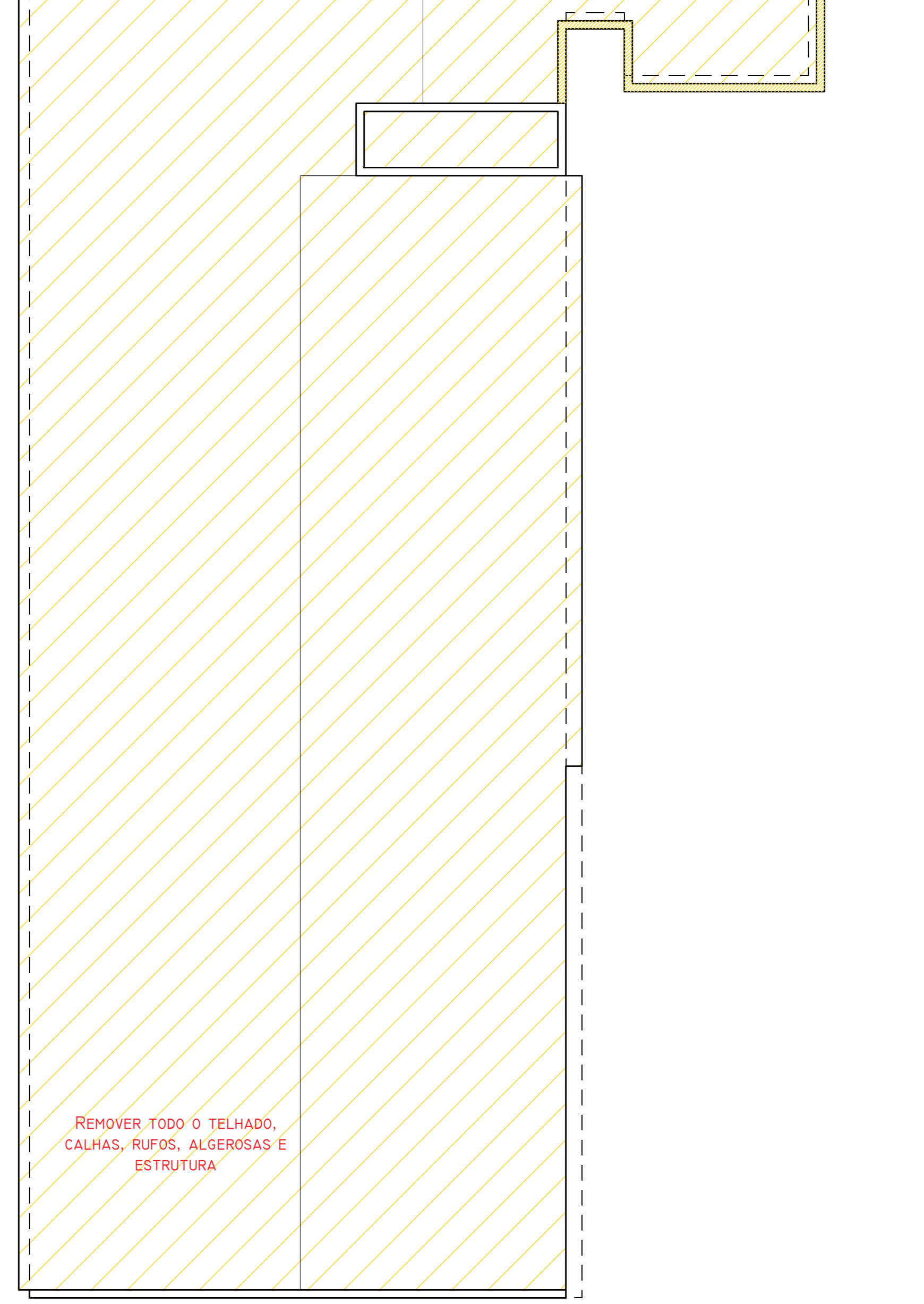
PLANTA DE COBERTURA - A DEMOLIR ESC 1/75
