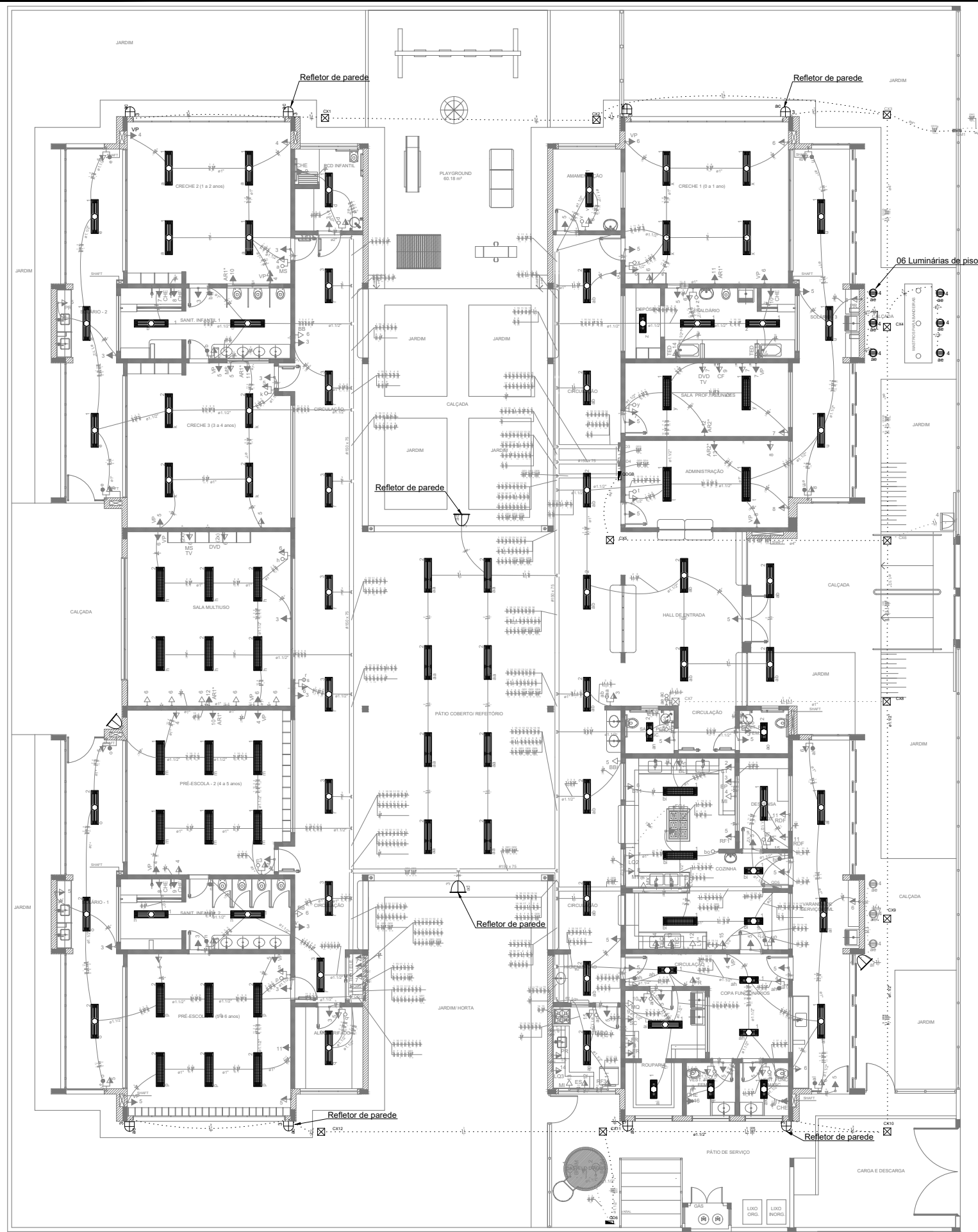
11 PLANTA BAIXA - ELÉTRICA ESCALA 1/200
