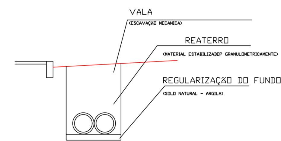
DETALHE DA VALA ASSENTAMENTO DA TUBULAÇÃO
