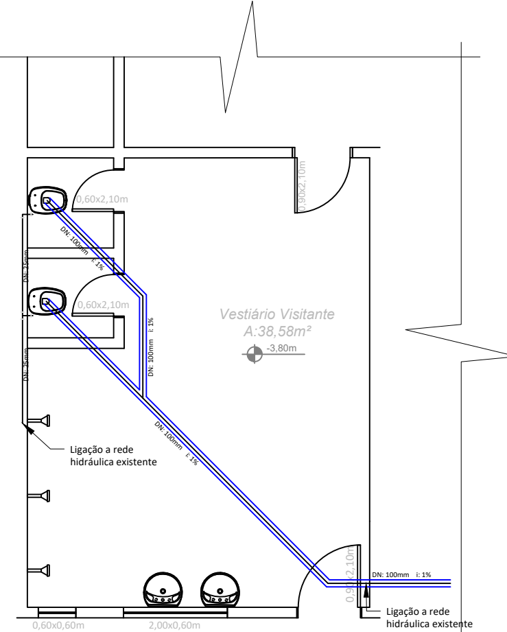
REDE HIDRÁULICA - VESTIÁRIO Esc: 1:50
