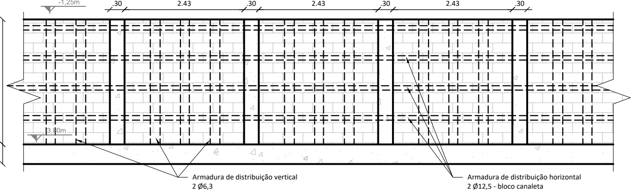
DETALHAMENTO MURO DE ARRIMO Esc: 1:75
