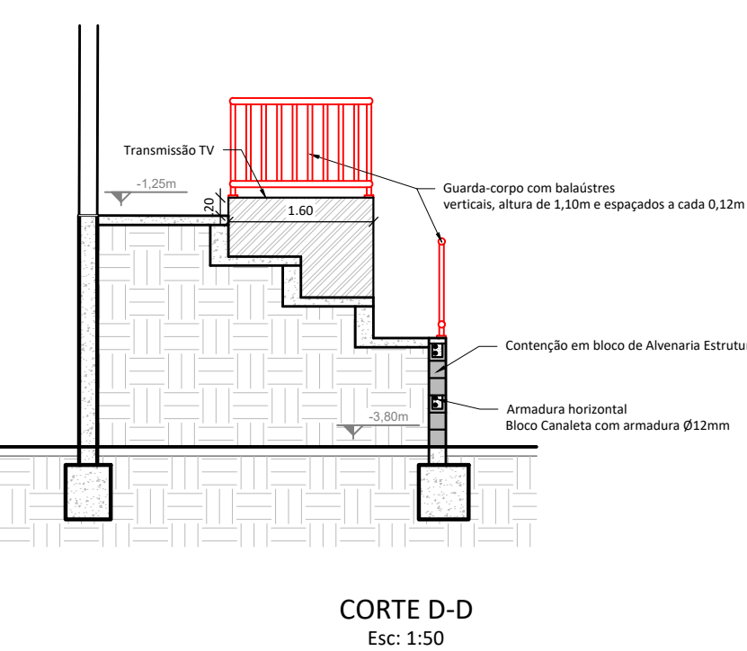
CORTE D-D Esc: 1:50
