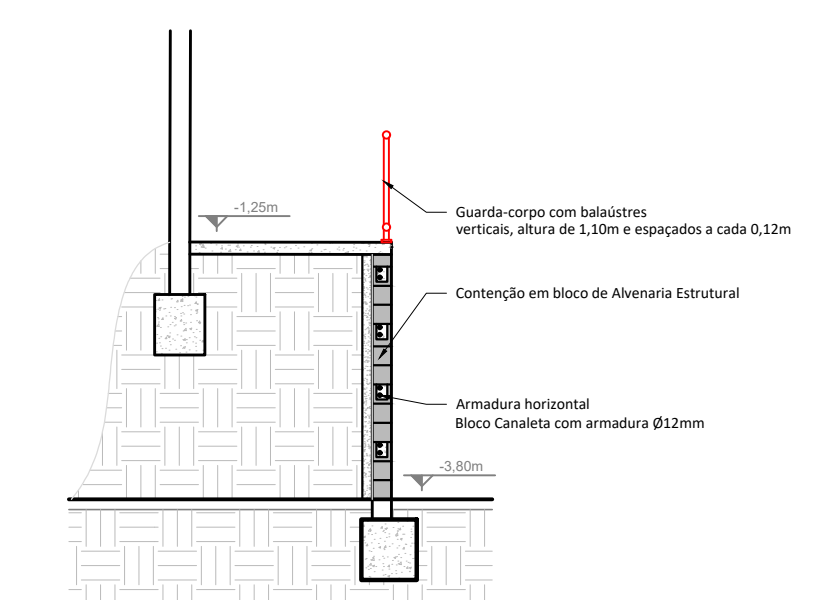
CORTE E-E Esc: 1:50
