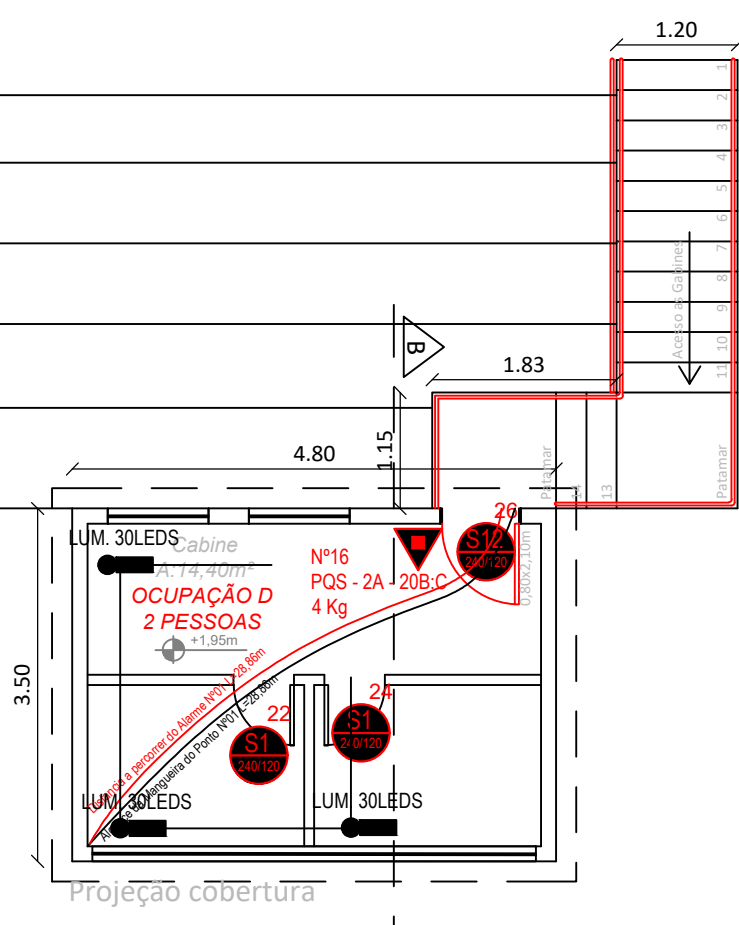
PPCL - CABINES RÁDIO Esc: 1:50
