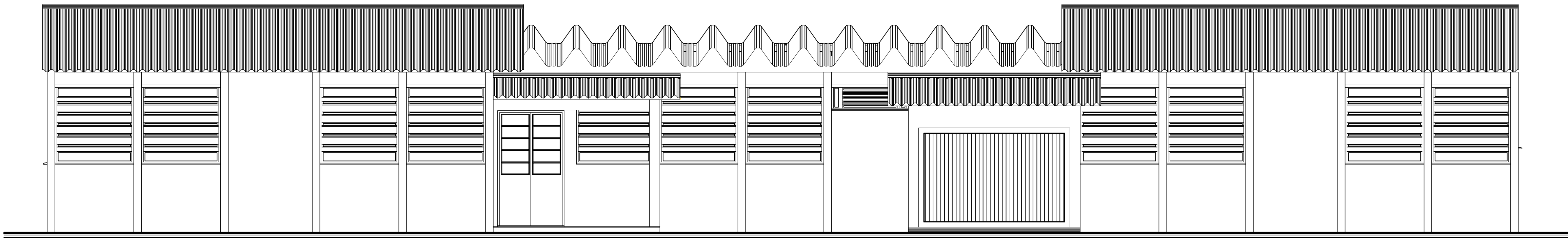
FACHADA FRONTAL
