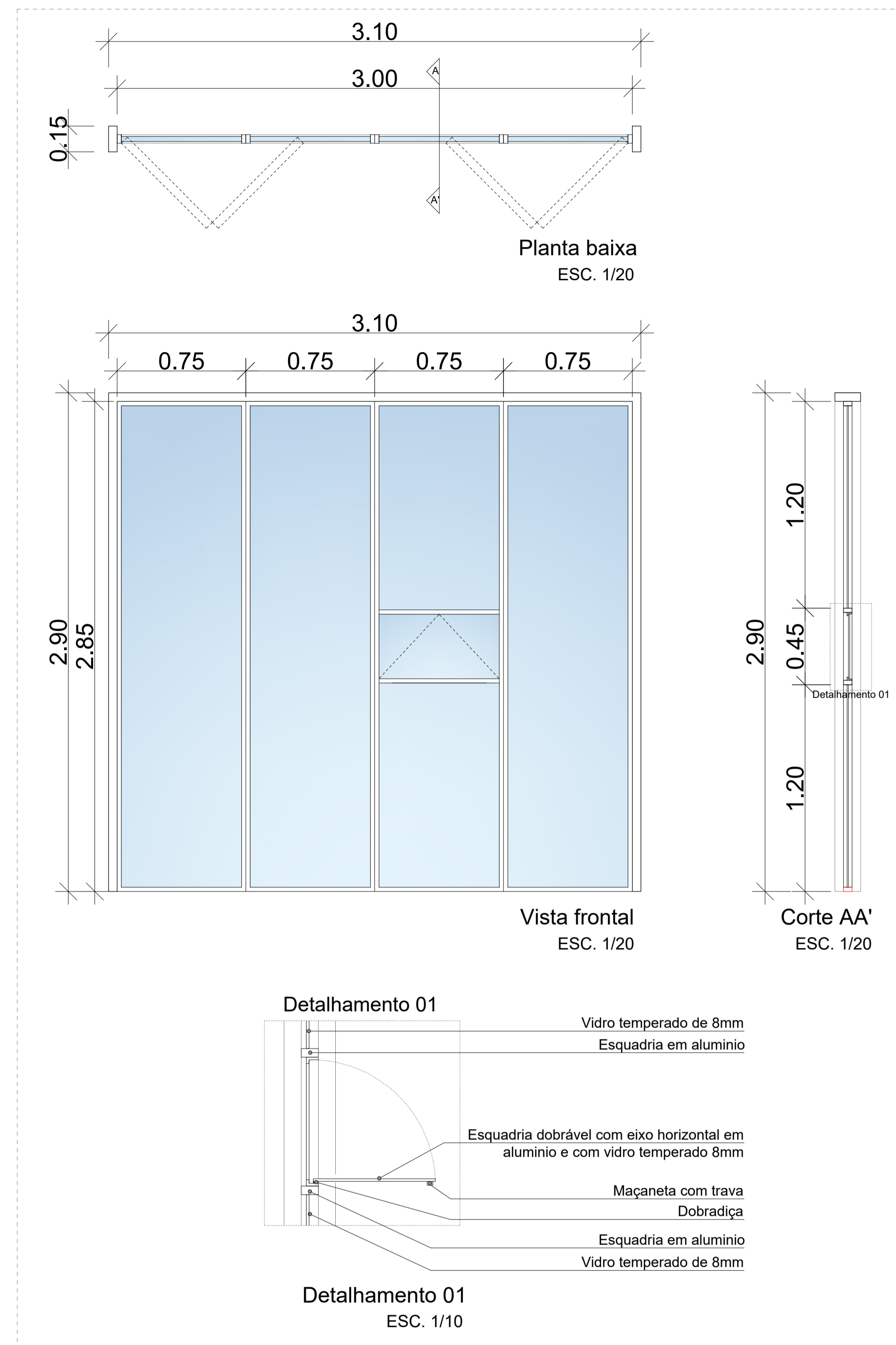
5 DETALHAMENTO PORTA ENTRADA ESC. INDICADA
