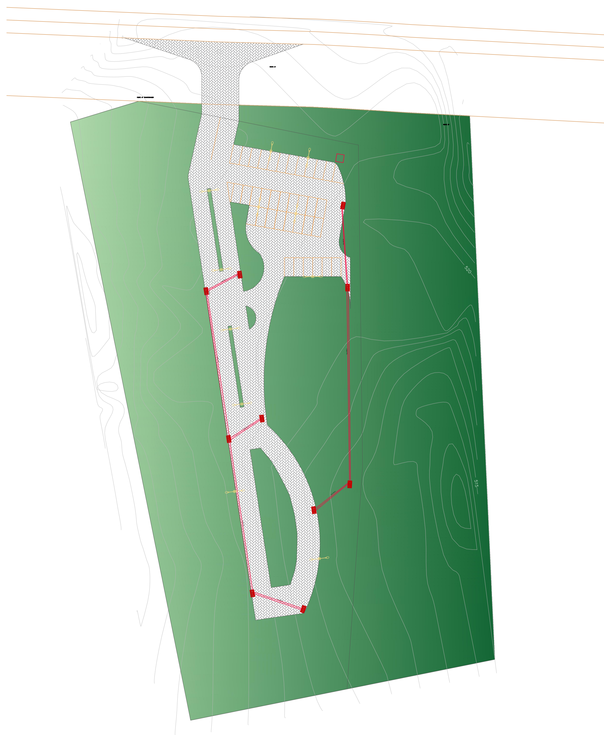
1 IMPLANTAÇÃO INFRAESTRUTURA ESCALA: 1 : 500
