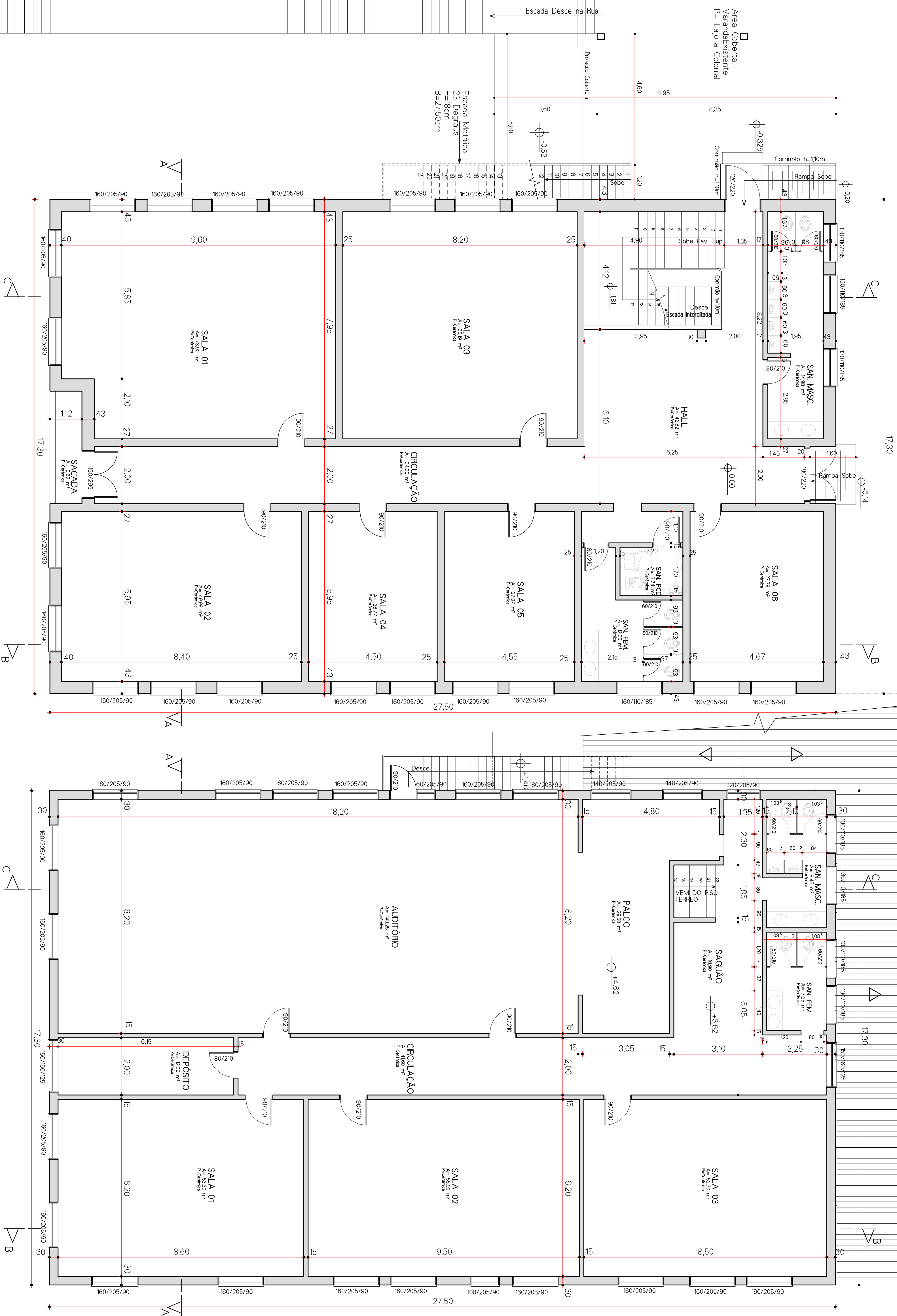
PLANTA BAIXA PAV. 2º PAVIMENTO FUTURO COM AS MELHORIAS
