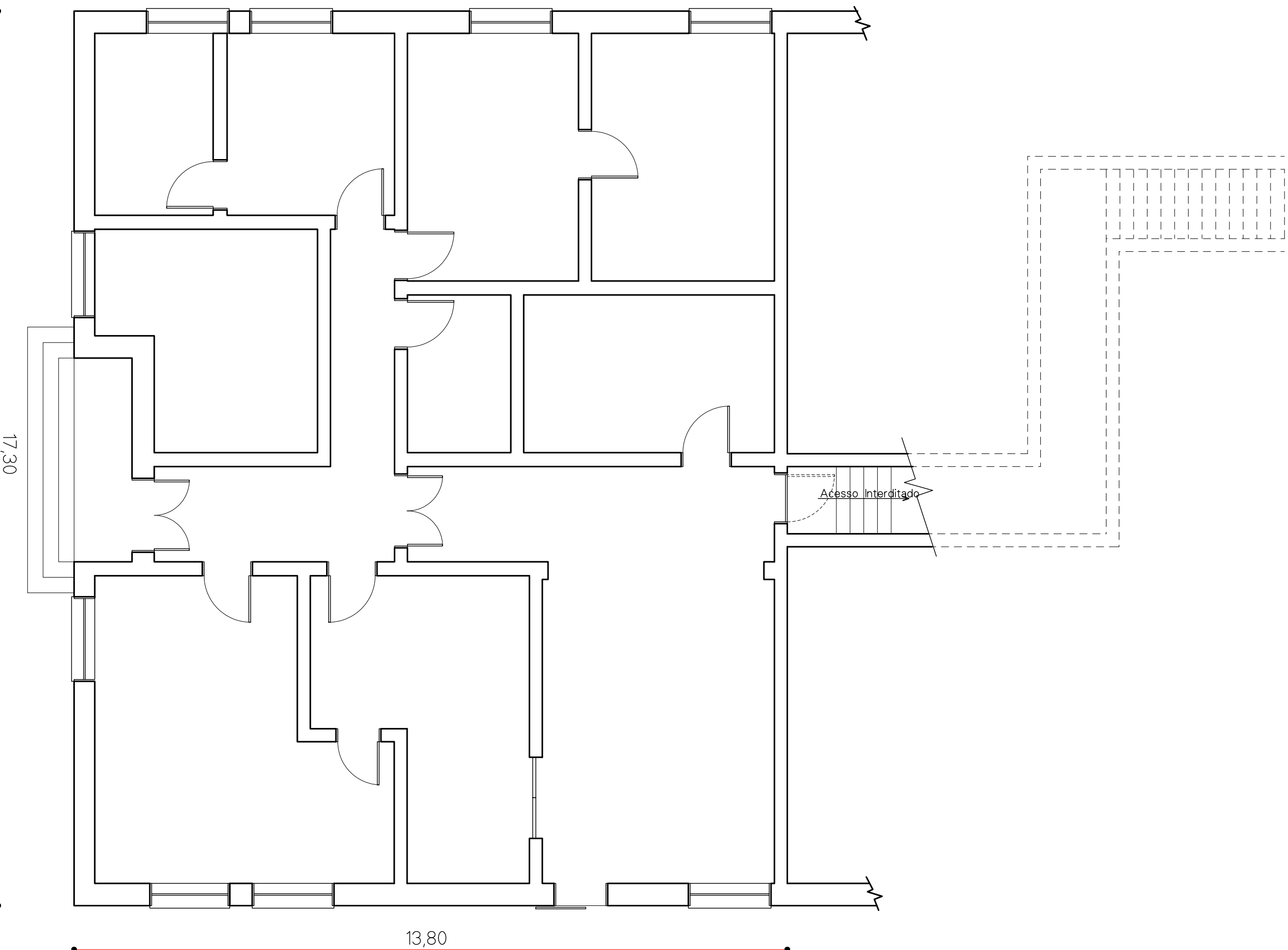
PLANTA BAIXA PAV. TERREO ATUAL
