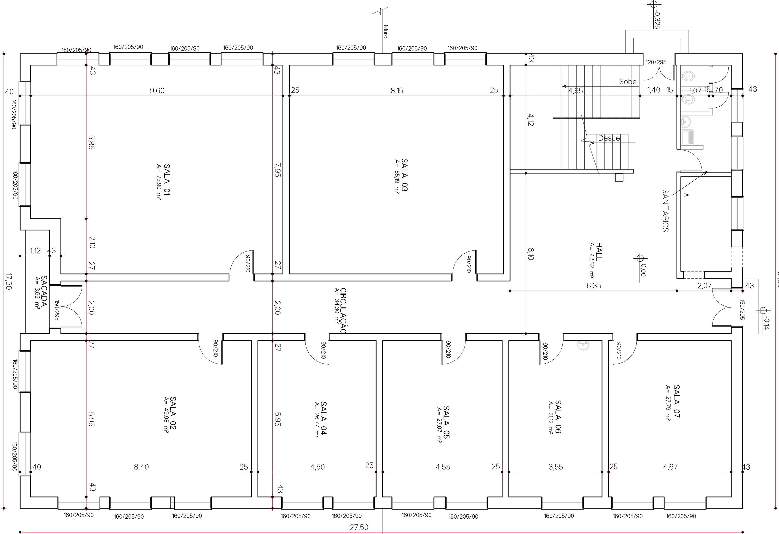
PLANTA BAIXA 2º PAVIMENTO ATUAL
