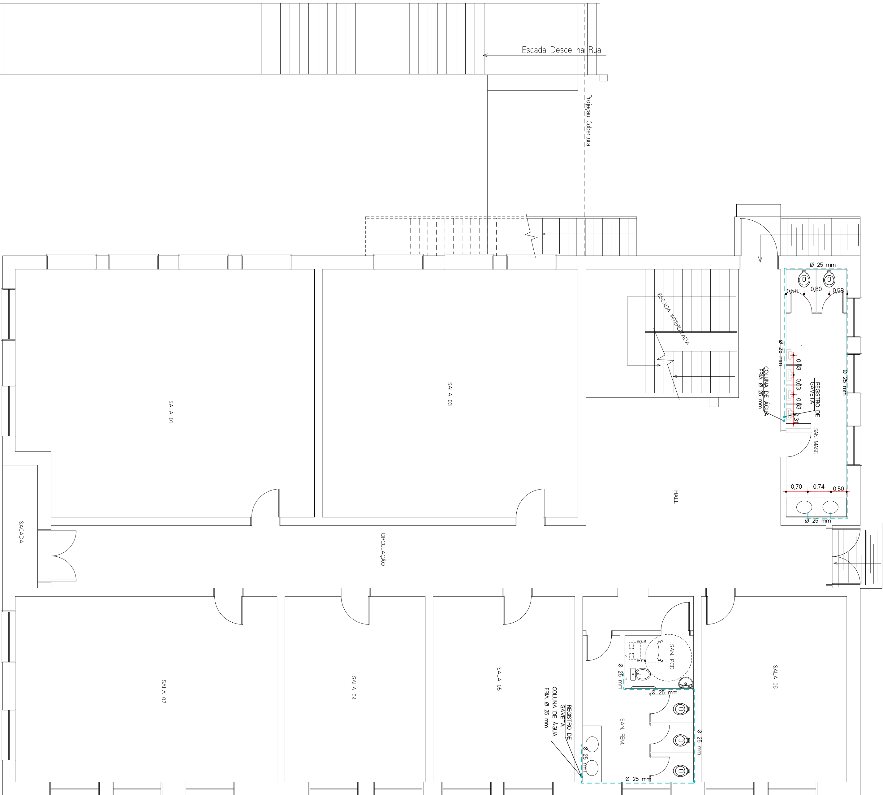
PLANTA BAIXA 2º PAVIMENTO COM AS MELHORIAS
