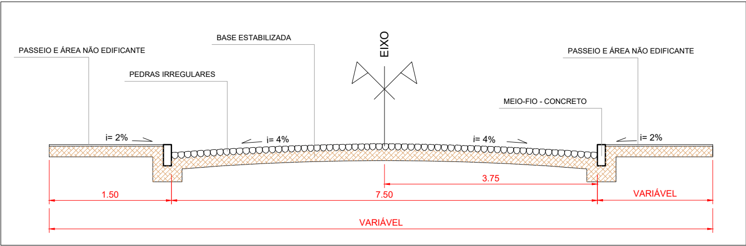
Seção transversal
