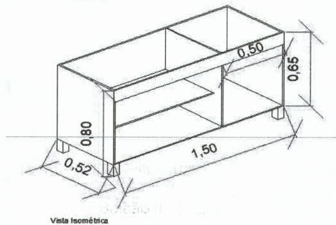
Balcão de cozinha auxiliar
