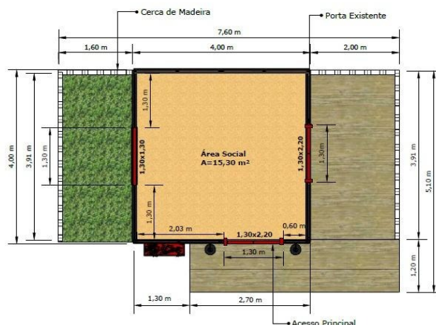
PLANTA BAIXA TÉRREO ESCALA 1:50
