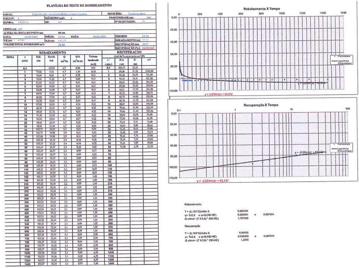
Figura 9. Modelo de planilha para realização do teste de vazão com apresentação dos resultados em gráfico com escala logarítmica e equação da reta.
