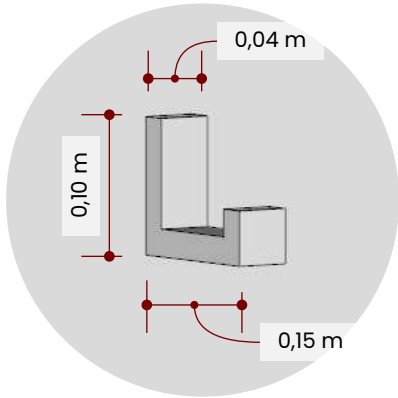
DET.01 - SUPORTE ACERVO
