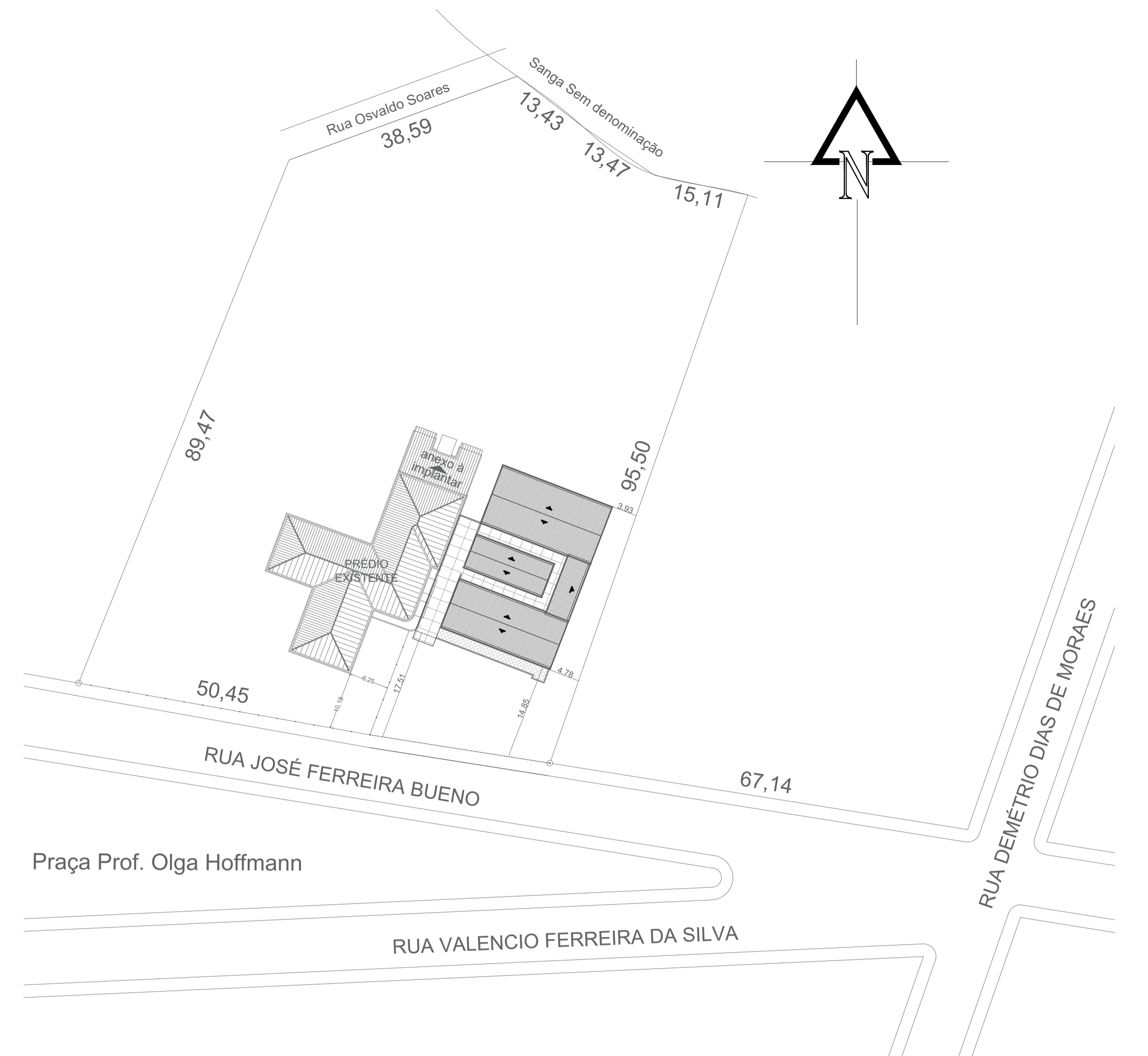
2 PLANTA DE SITUAÇÃO Área total: 7.000m 2 1 : 500
