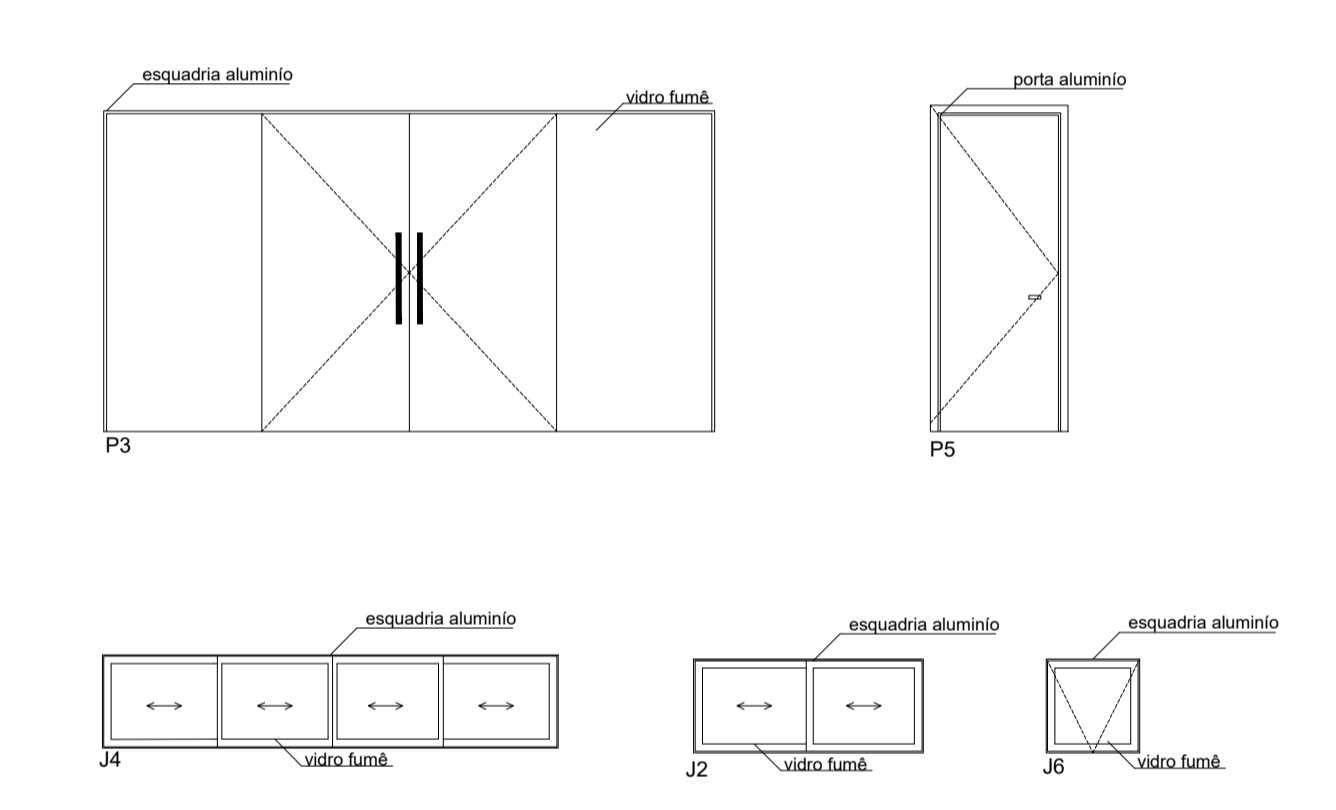
2 DETALHES 1 : 50
