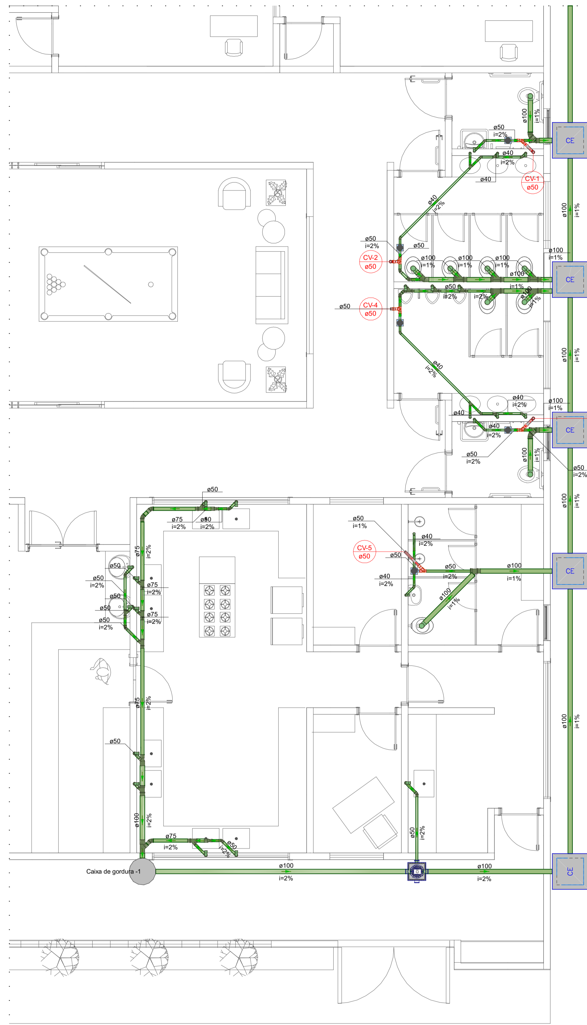
Detalhe SAN-1 Escala 1:50
