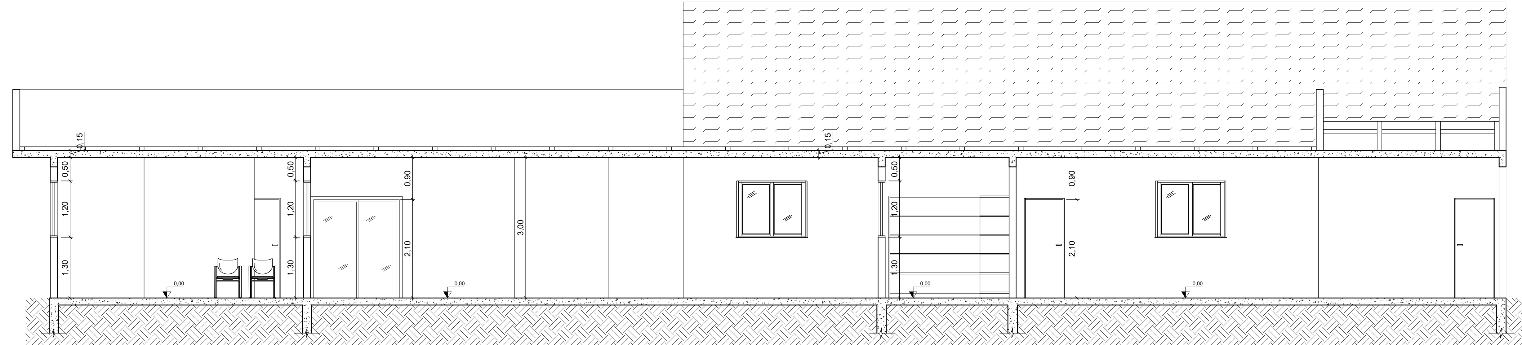
CORTE AA'
