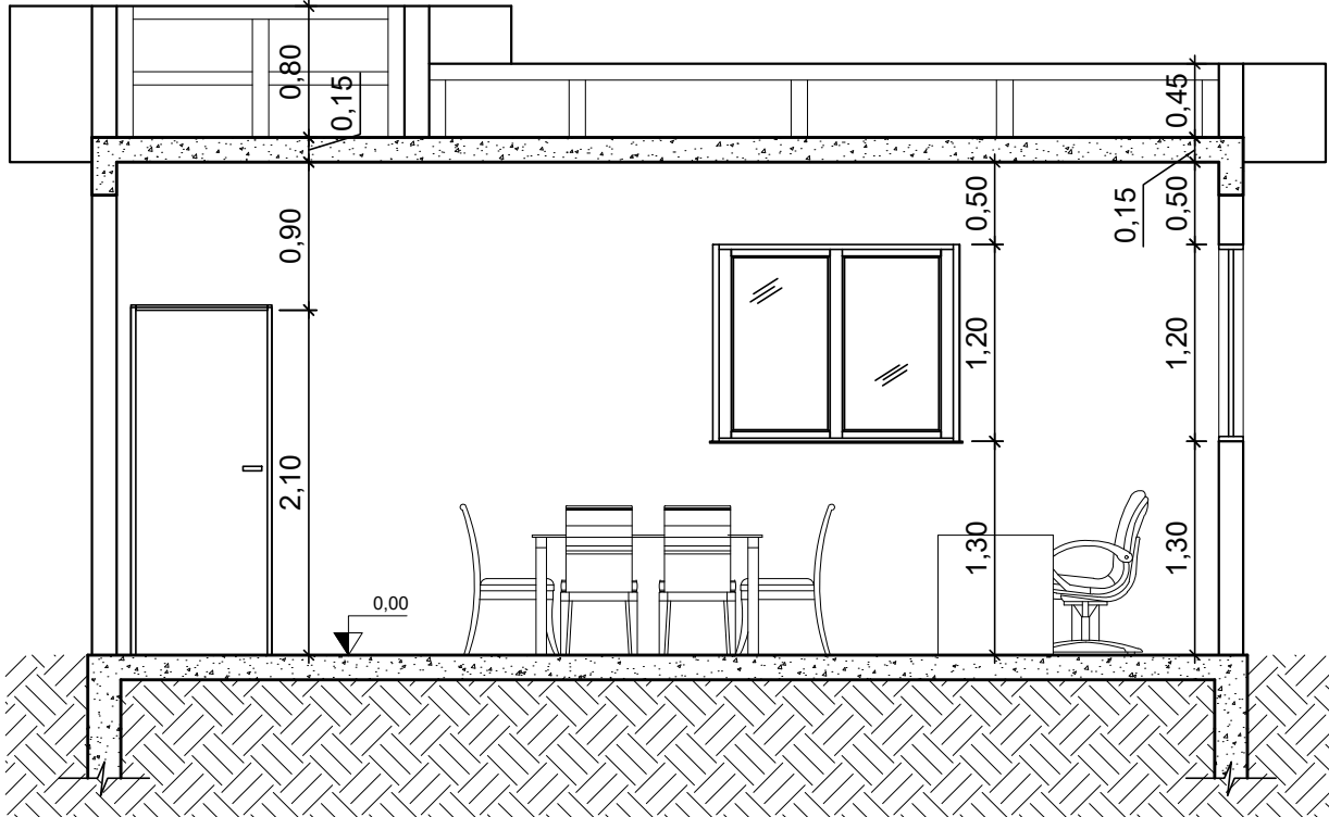
CORTE DD'
