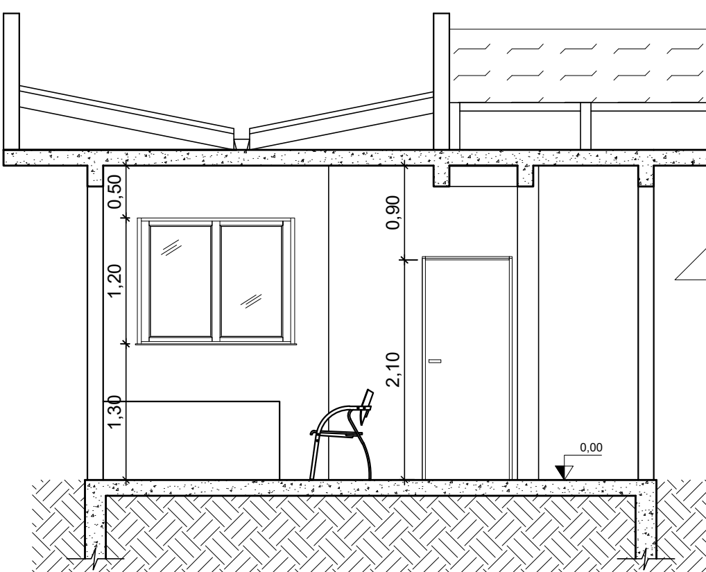
CORTE BB'
