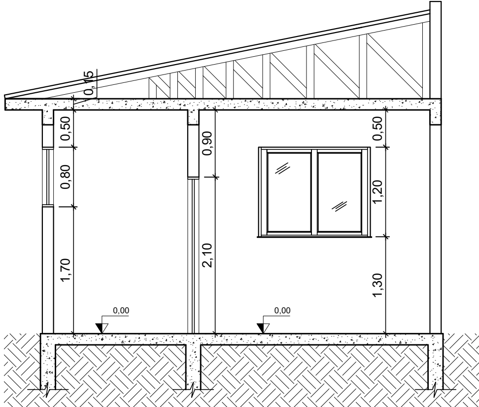
CORTE CC'
