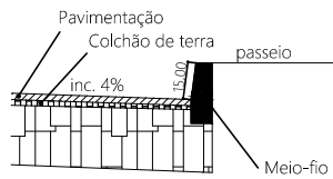
SEÇÃO TIPO PAVIMENTO ESC. 1/100
