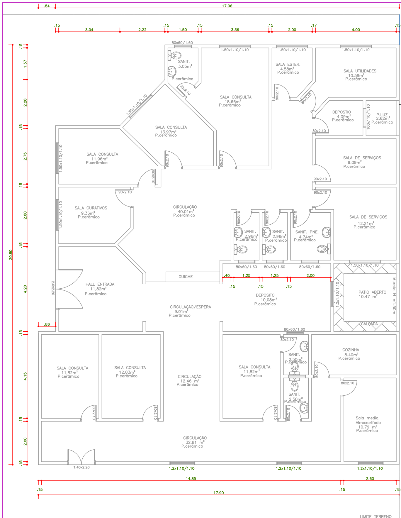
PLANTA DE SITUAÇÃO ATUAL PLANTA BAIXA, escala: 1/100 ÁREA: 340,99m 2
