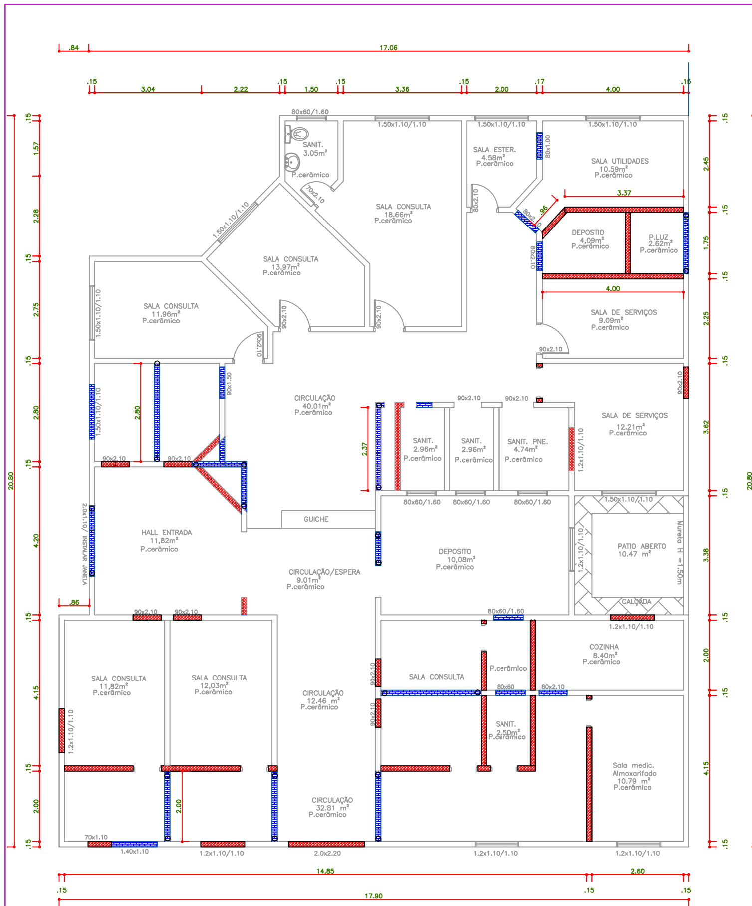
PAREDES A RETIRAR/EXECUTAR PLANTA BAIXA, escala: 1/100 ÁREA: 340,99m2
