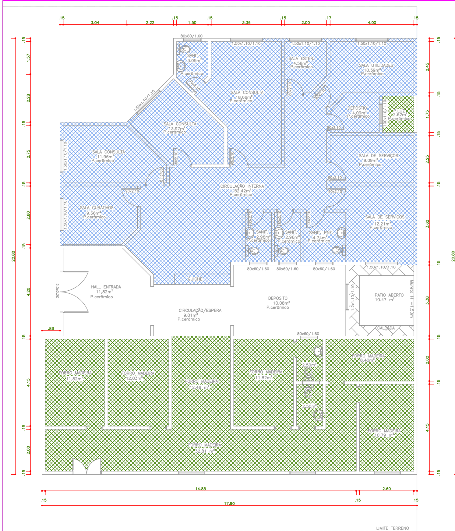
PLANTA DE FORRO A RETIRAR PLANTA BAIXA, escala: 1/100 ÁREA: 340,99m 2
