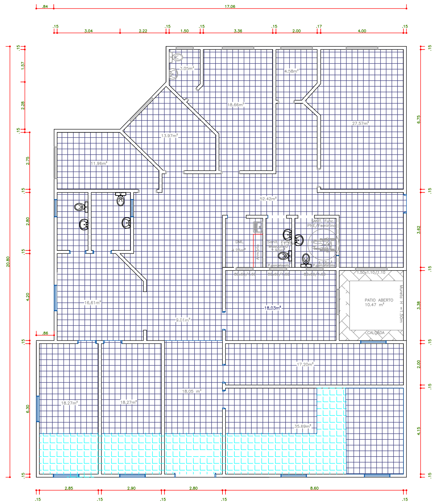
PLANTA DE PISO NOVO PLANTA BAIXA, escala: 1/100 ÁREA: 340,99m 2
