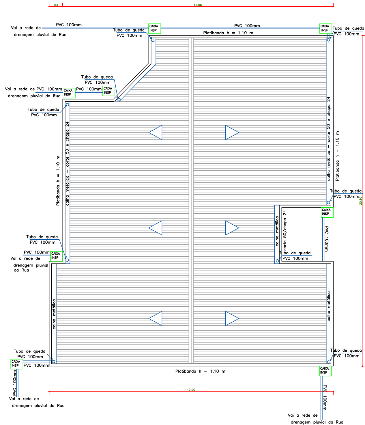
PLANTA DE COBERTURA/DRENAGEM PLUVIAL PLANTA DE DESCIDAS, escala: 1/125 ÁREA: 340,99m 2
