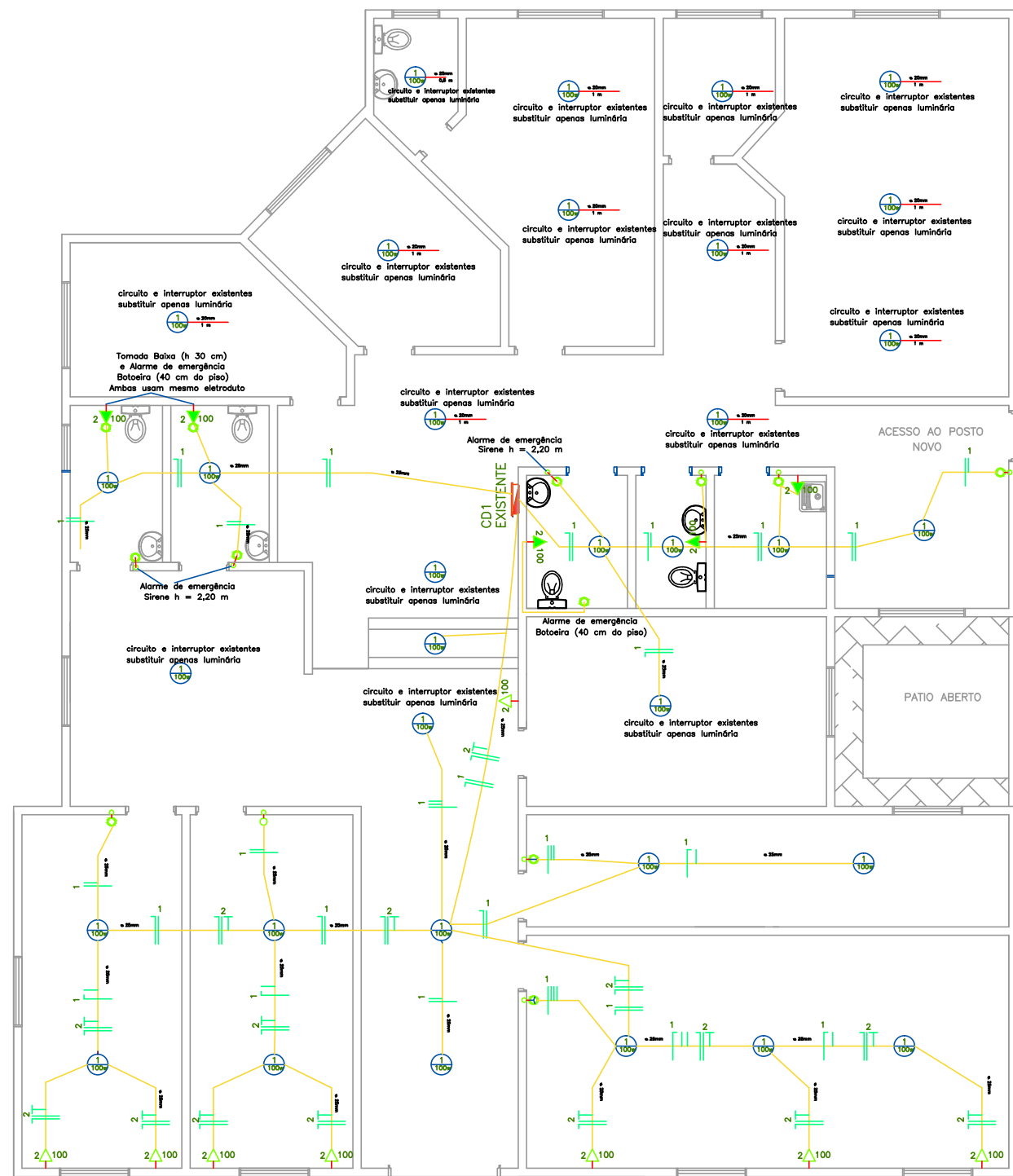
PROJETO ELETRICO PLANTA DE ADEQUAÇÕES, escala: 1/100 ÁREA: 340,99m 2
