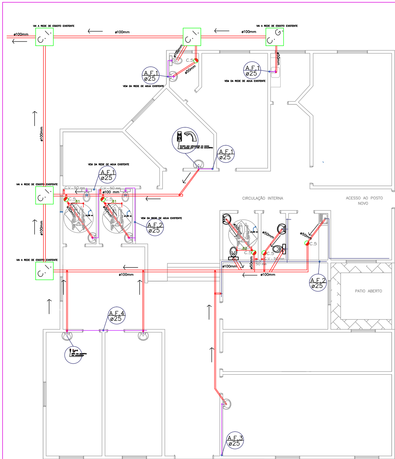
PROJETO HIDROSSANITÁRIO PLANTA BAIXA, escala: 1/100 ÁREA: 340,99m 2
