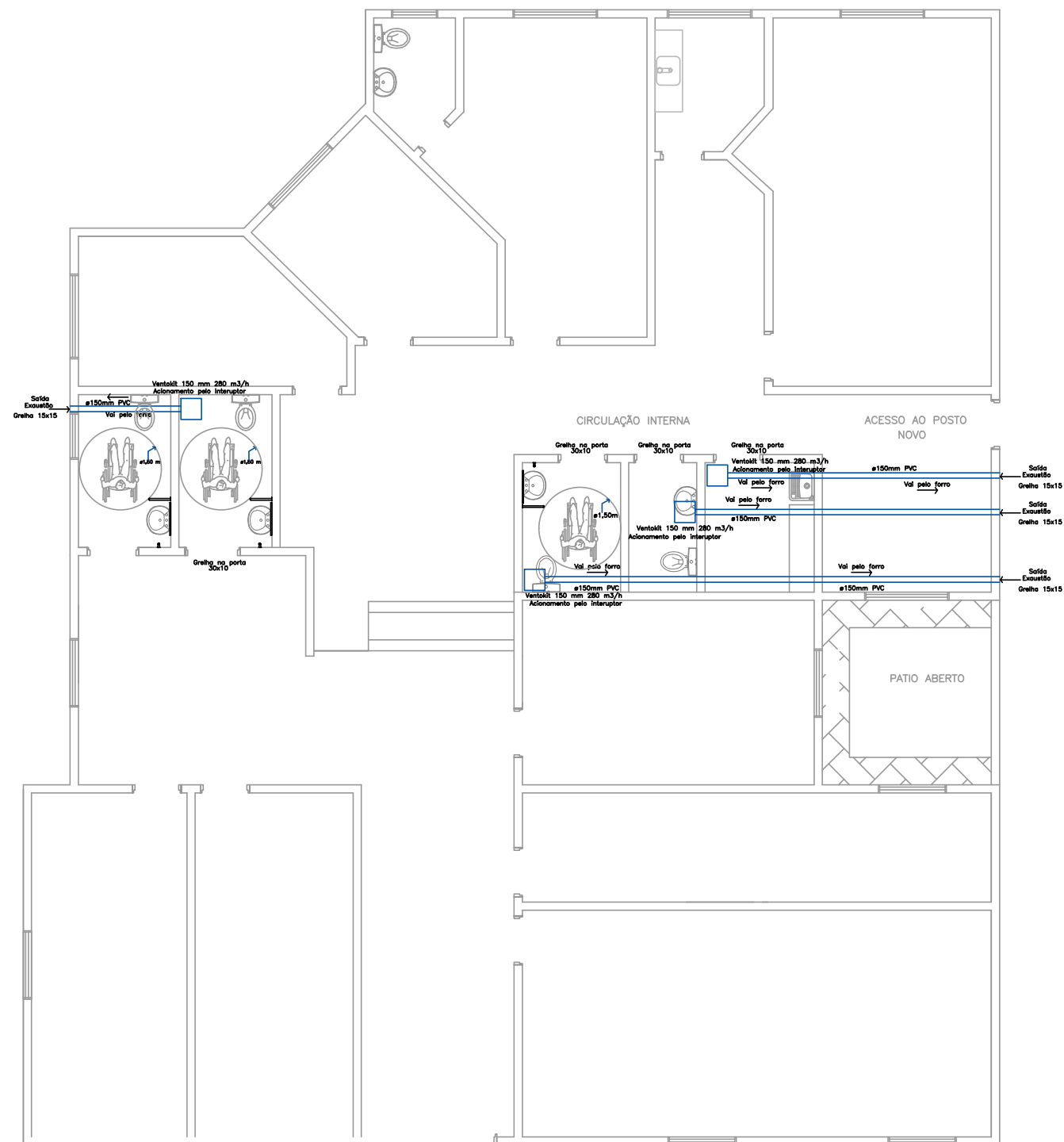
PROJETO RENIVAÇÃO DE AR/EXAUSTÃO PLANTA BAIXA, escala: 1/100 ÁREA: 340,99m2
