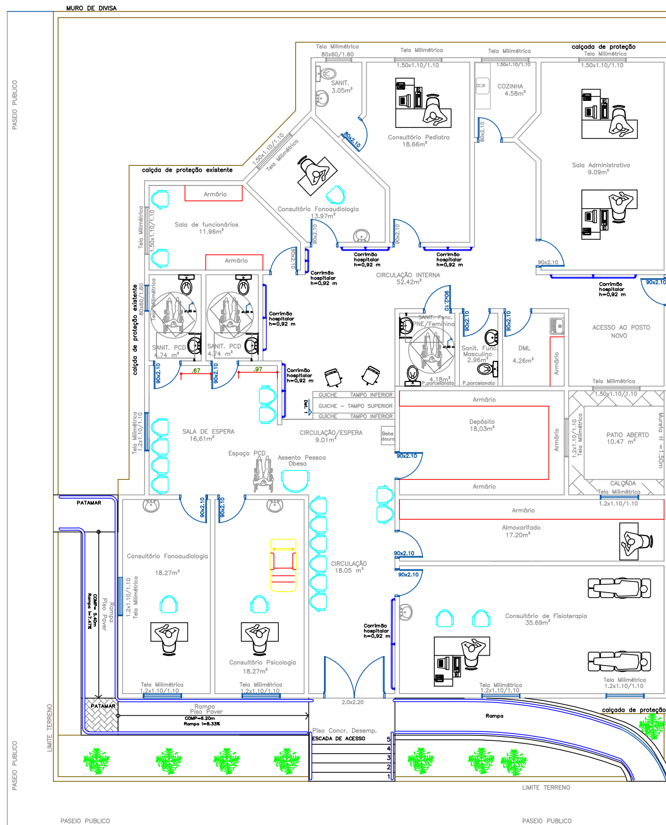
SITUAÇÃO FINAL/PRETENDIDA – PLANTA MOBILIADA ACESSO FRONTAL E LATERAL, escala: 1/125 ÁREA: 340,99m 2
