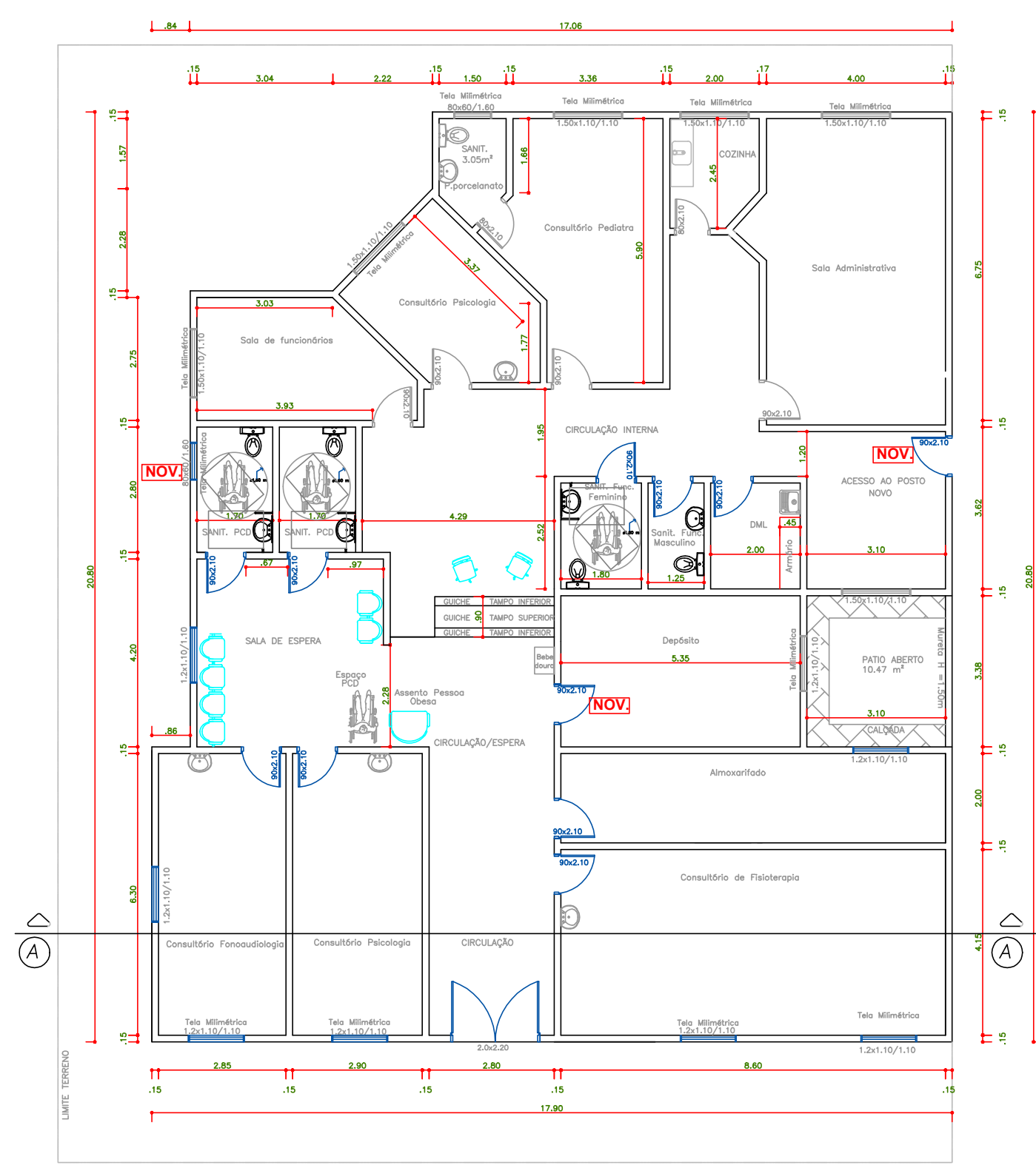
PLANTA BAIXA COTADA PLANTA BAIXA, escala: 1/100 ÁREA: 340,99m 2
