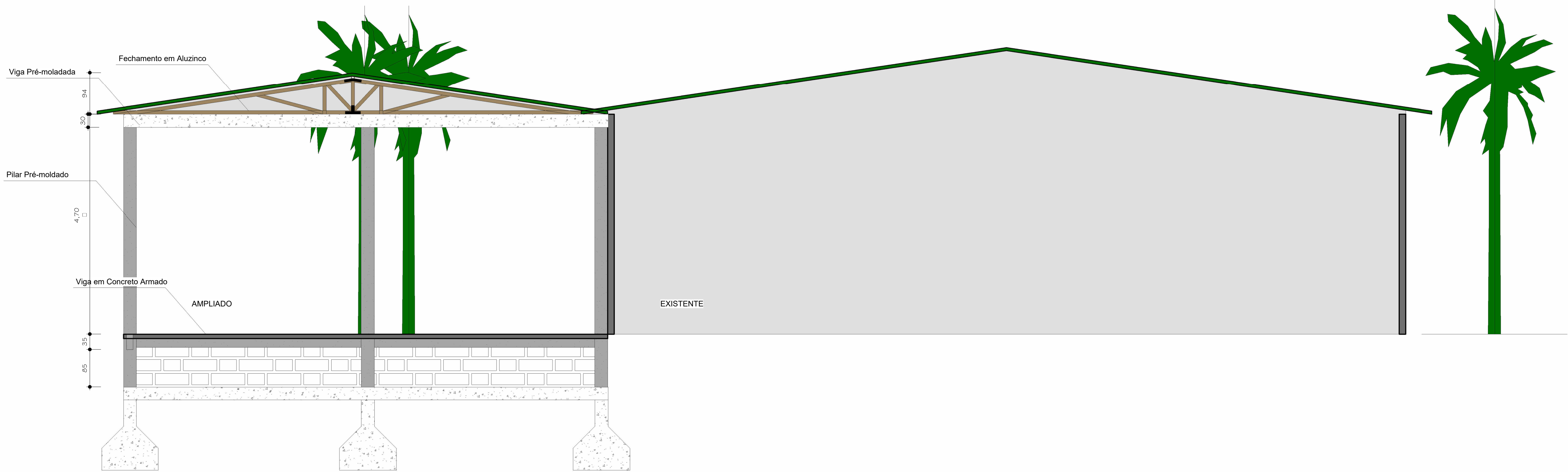
1 Corte AA 1 : 50
